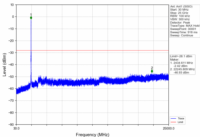
802.11n(HT40)_MCH_2437MHz_Ant1 (SISO)_NTNV
