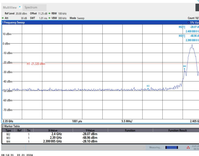
BLE_2M_Ant1_Low_2402
