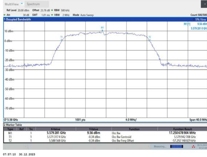
11A_Ant2_5580
