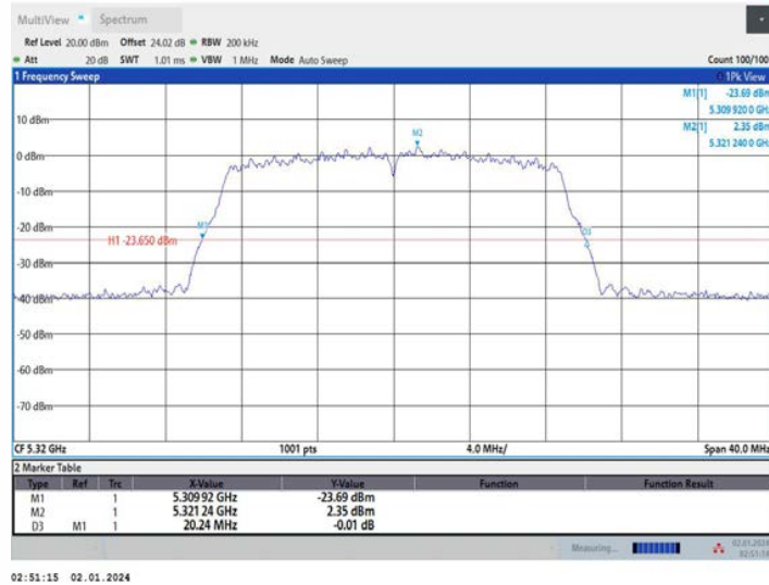
11AC20MIMO_Ant2_5320
