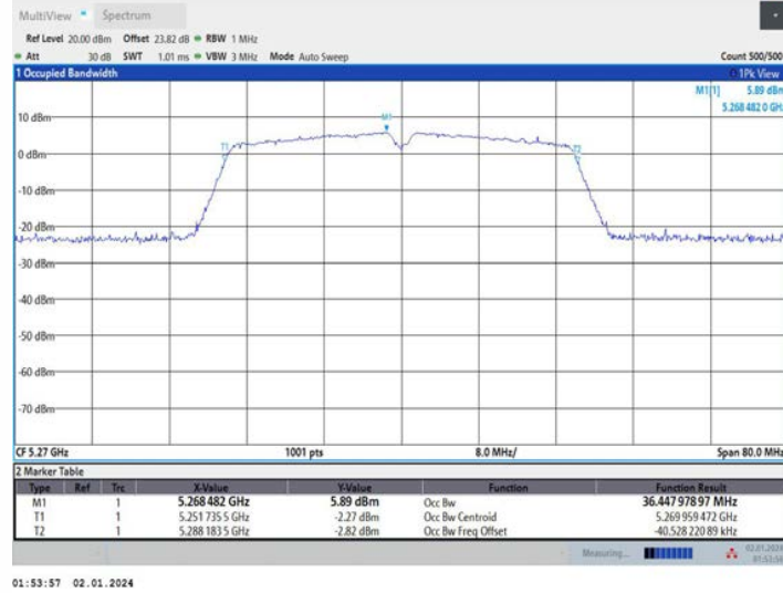
11N40MIMO_Ant2_5270
