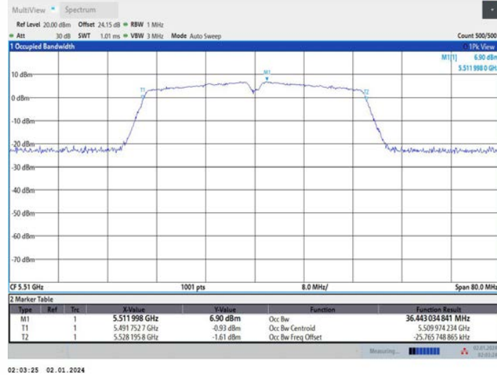
11N40MIMO_Ant2_5510
