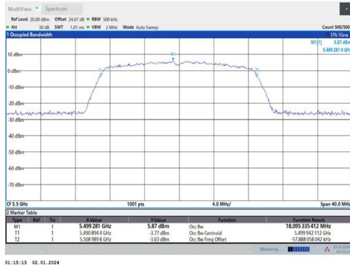
11N20MIMO_Ant2_5500
