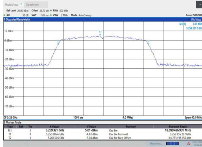
11N20MIMO_Ant2_5260
