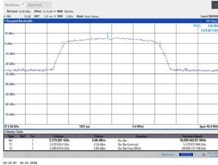
11AC20MIMO_Ant2_5580
