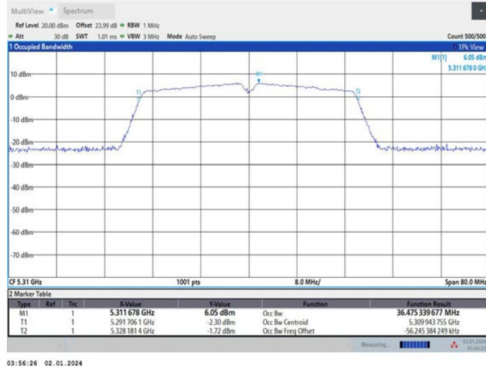
11AC40MIMO_Ant2_5310
