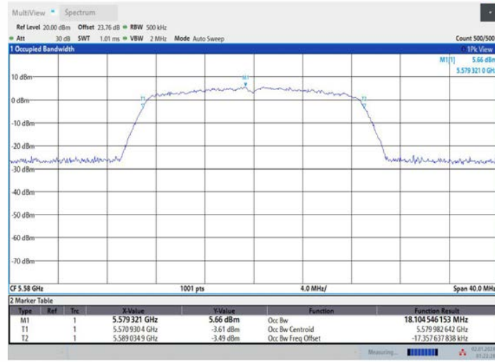
11N20MIMO_Ant2_5580
