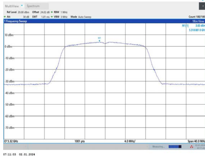
11A_Ant2_5320
