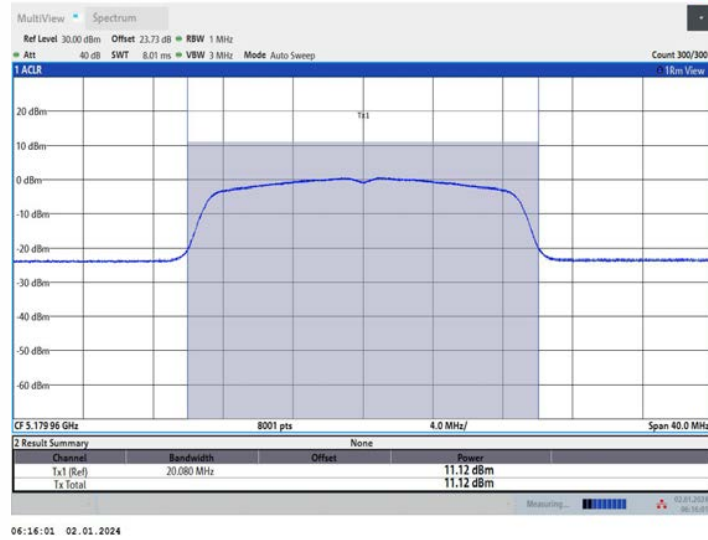
11AC20MIMO_Ant2_5180
