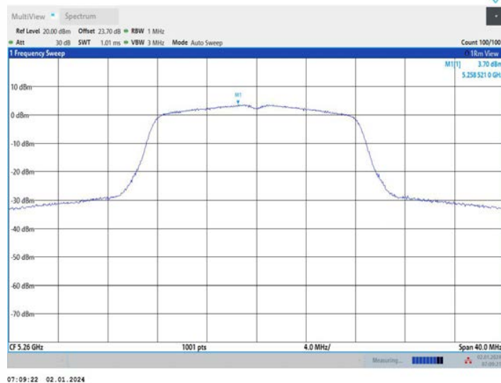
11A_Ant2_5260
