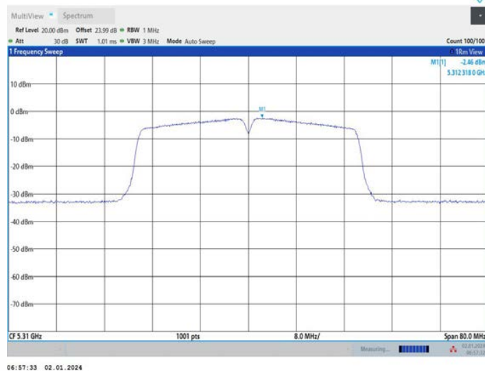
11N40MIMO_Ant2_5310
