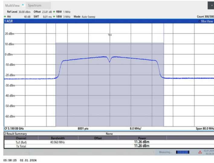
11AC40MIMO_Ant2_5190
