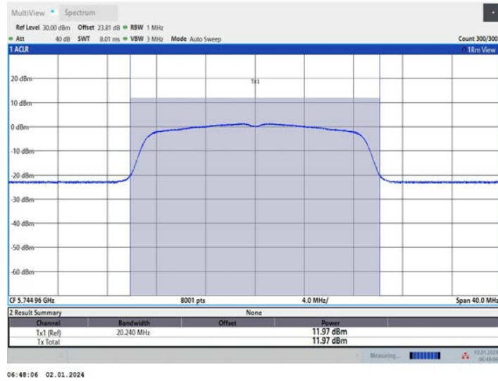
11N20MIMO_Ant2_5745
