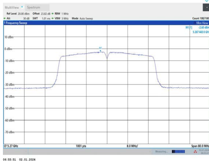
11N40MIMO_Ant2_5270
