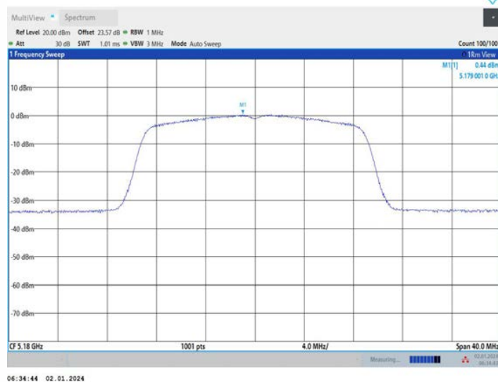
11N20MIMO_Ant2_5180
