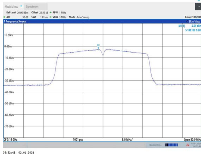
11N40MIMO_Ant2_5190
