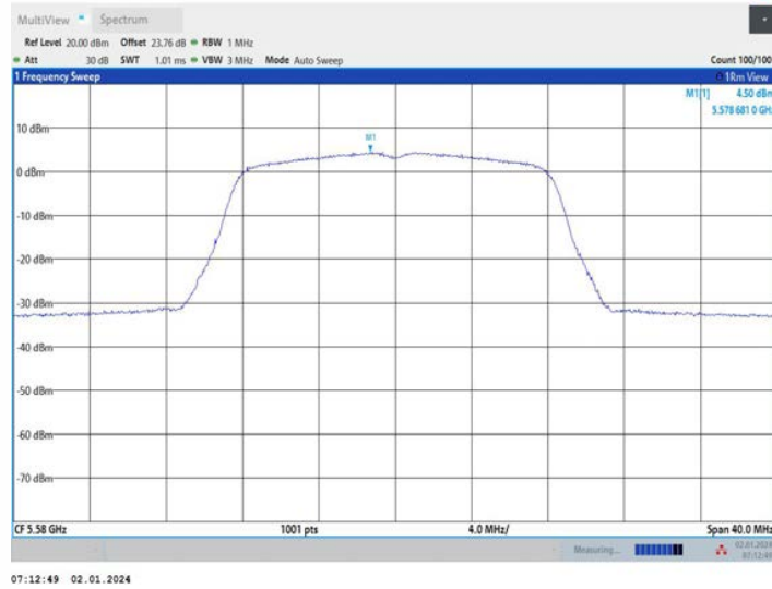
11A_Ant2_5580
