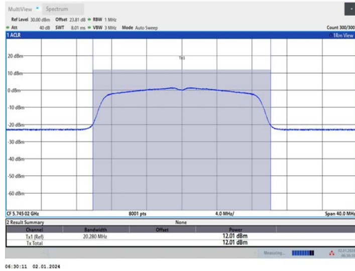
11AC20MIMO_Ant2_5745
