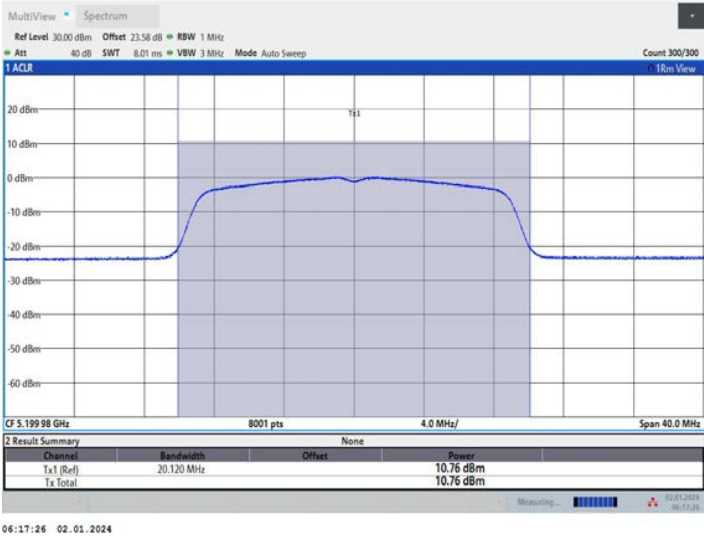
11AC20MIMO_Ant2_5200
