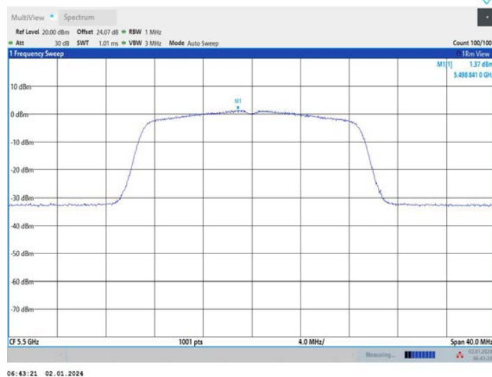
11N20MIMO_Ant2_5500
