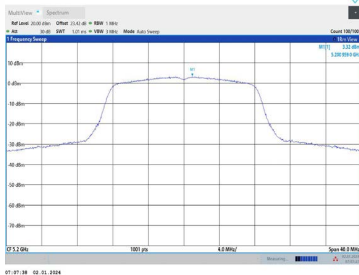
11A_Ant2_5200
