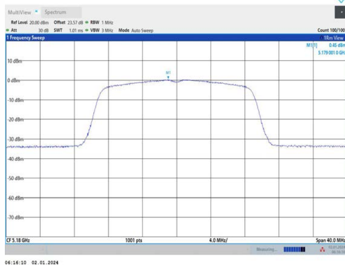
11AC20MIMO_Ant2_5180
