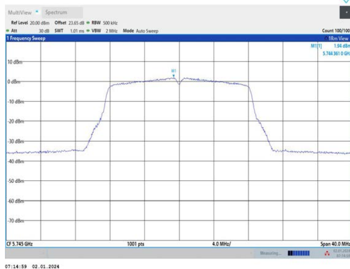
11A_Ant2_5745
