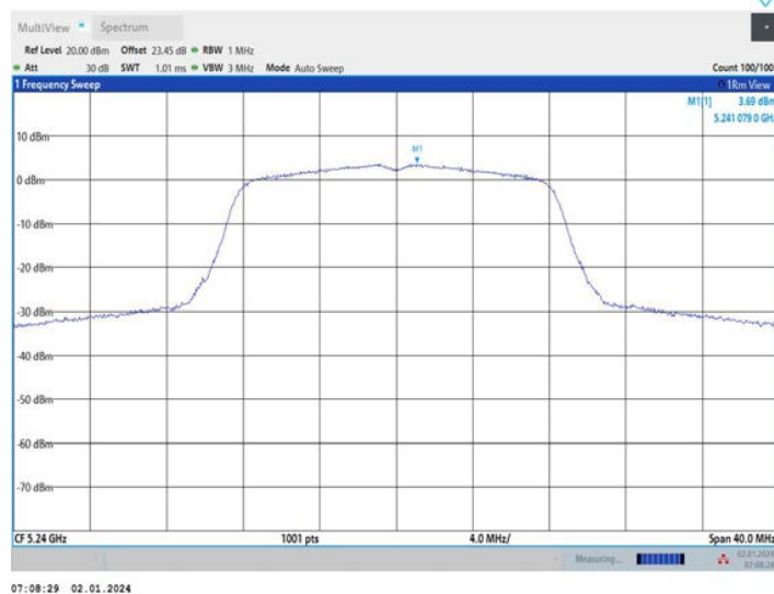
11A_Ant2_5240
