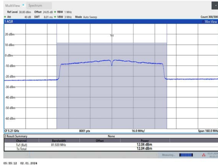
11AC80MIMO_Ant2_5210
