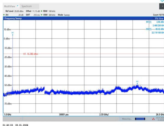
BLE_1M_Ant1_2480_1000~26500
