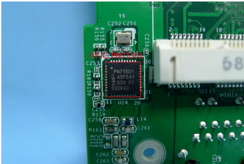
(21) EUT Photo
