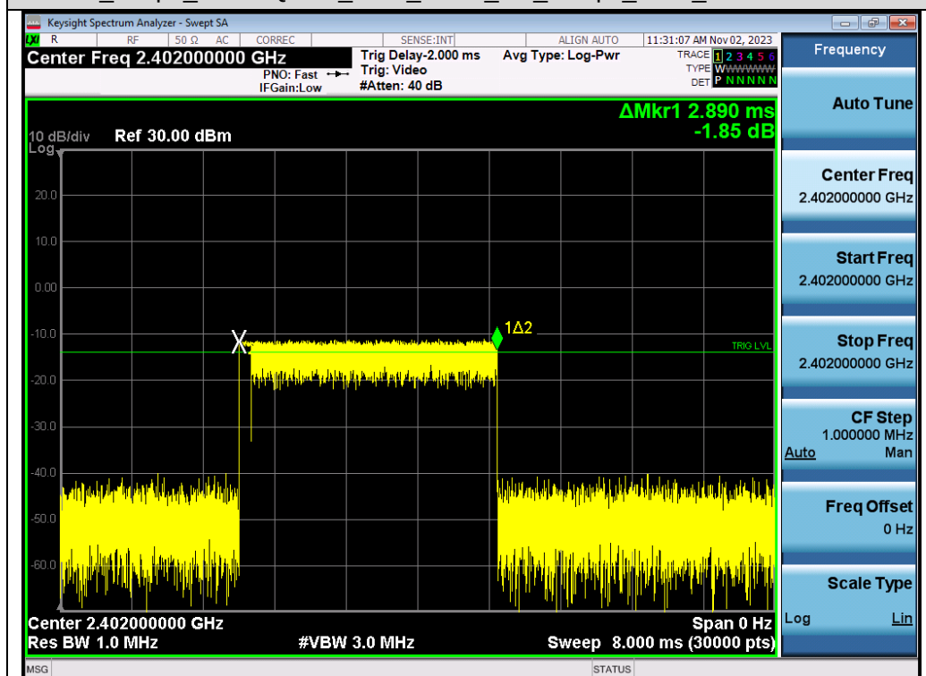
Test_Graph_π /4-DQPSK_HOP_ANT1_NA_1Mbps_2402_Time per Burst
