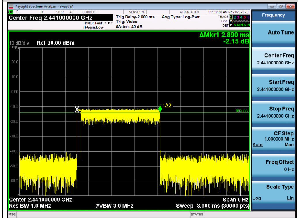
Test_Graph_π /4-DQPSK_HOP_ANT1_NA_1Mbps_2441_Time per Burst
