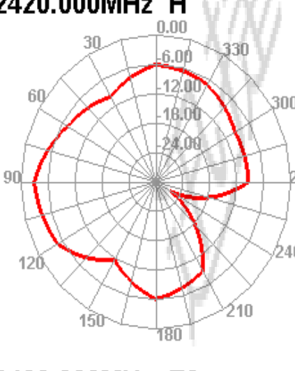
2420.000MHz H
