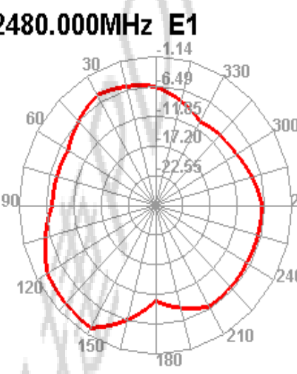
2480.000MHz
