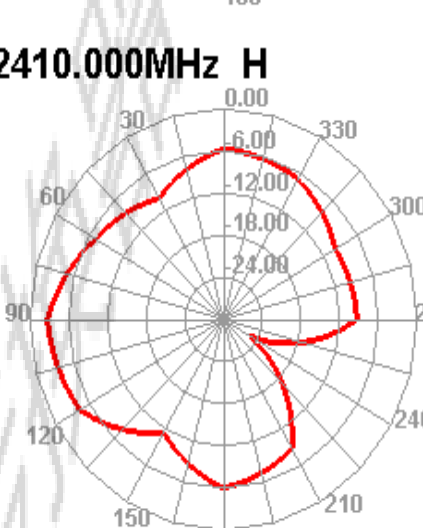
2410.000MHz H
