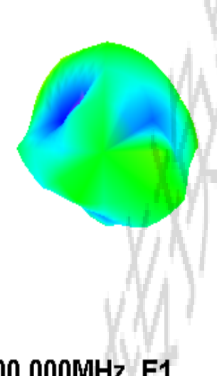
2490.000MHz E1
