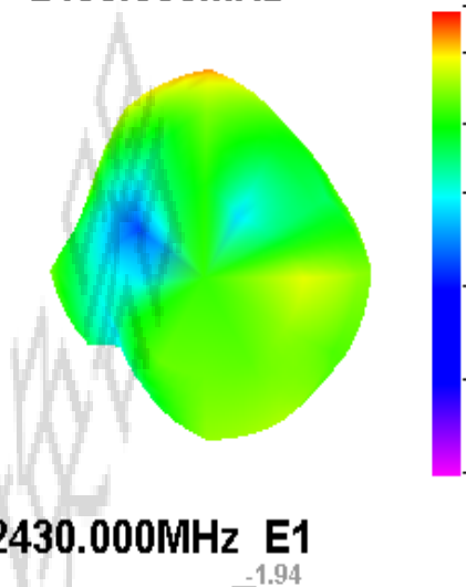
2430.000MHz
