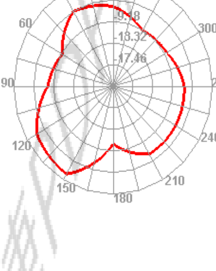
2500.000MHz
