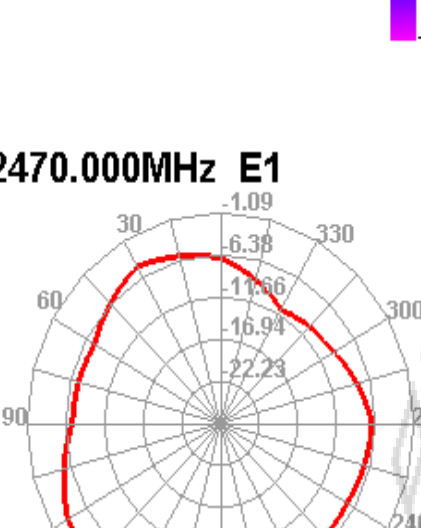
2470.000MHz
