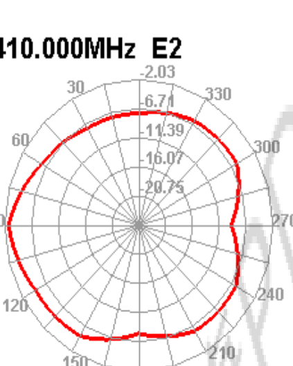
2410.000MHz E2
