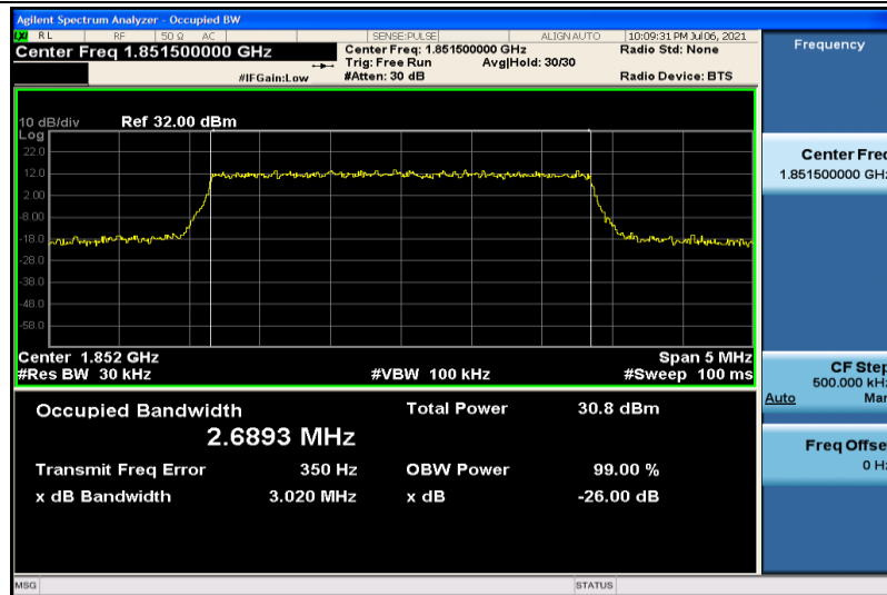
Band2-3MHz-QPSK-18615-15RB#0-2.6893
