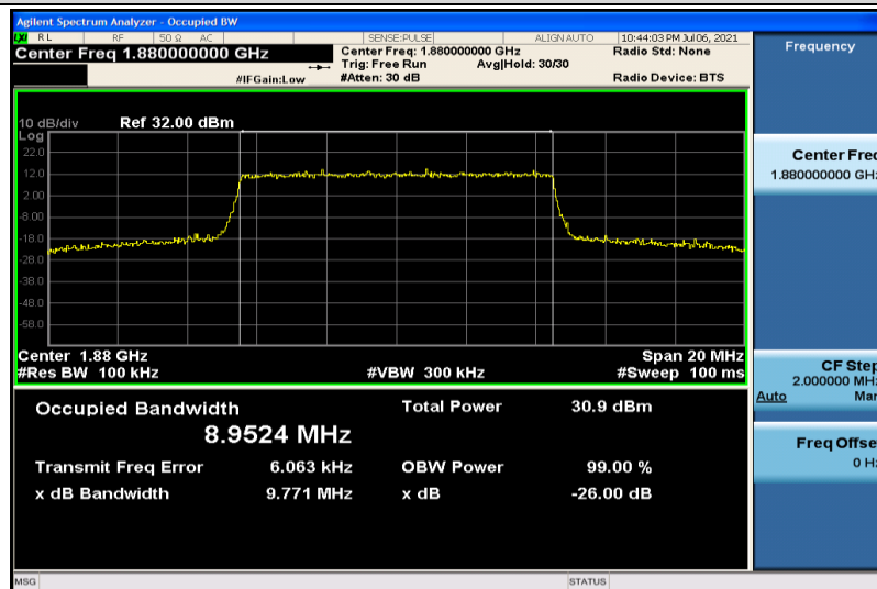
Band2-10MHz-QPSK-18900-50RB#0-8.9524
