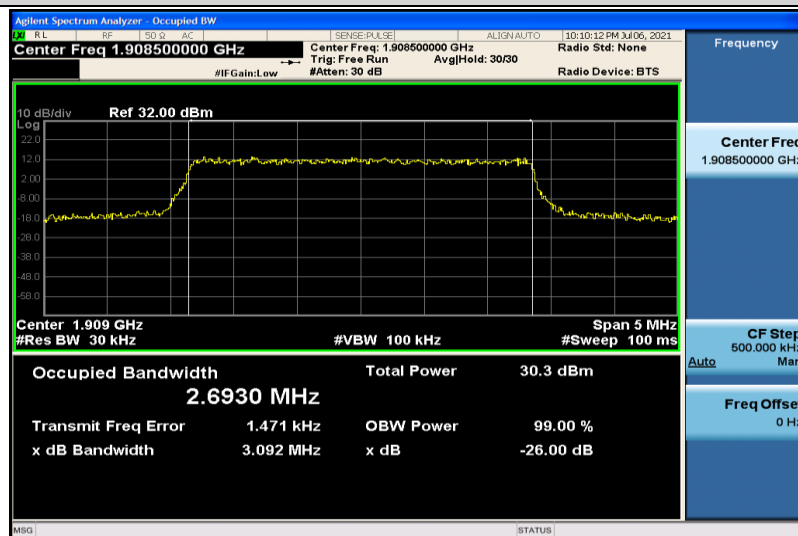
Band2-3MHz-QPSK-19185-15RB#0-2.6930
