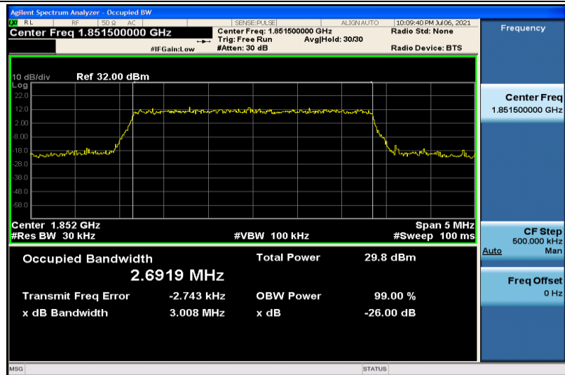
Band2-3MHz-16QAM-18615-15RB#0-2.6919
