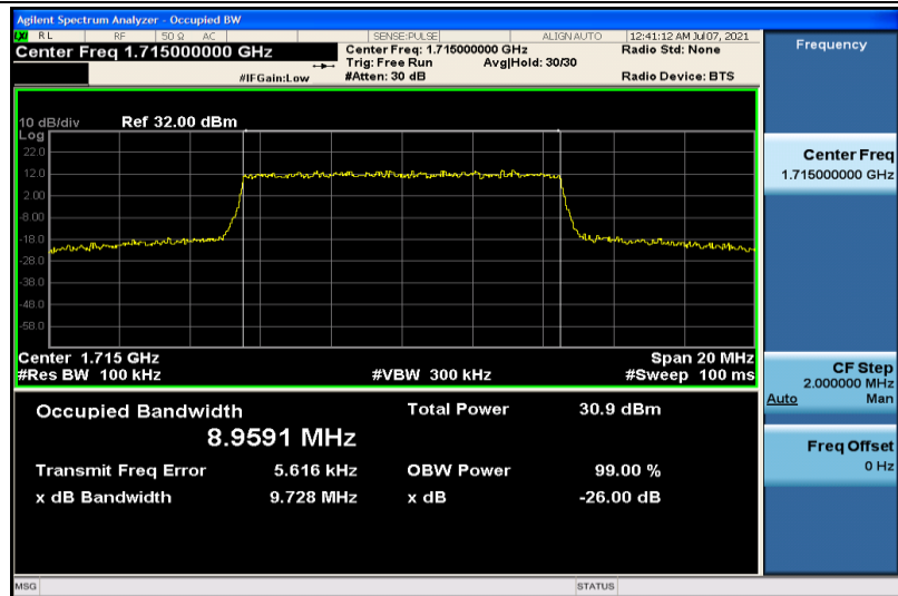
Band4-10MHz-QPSK-20000-50RB#0-8.9591
