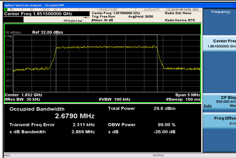
Band2-3MHz-QPSK-18615-15RB#0-2.6790
