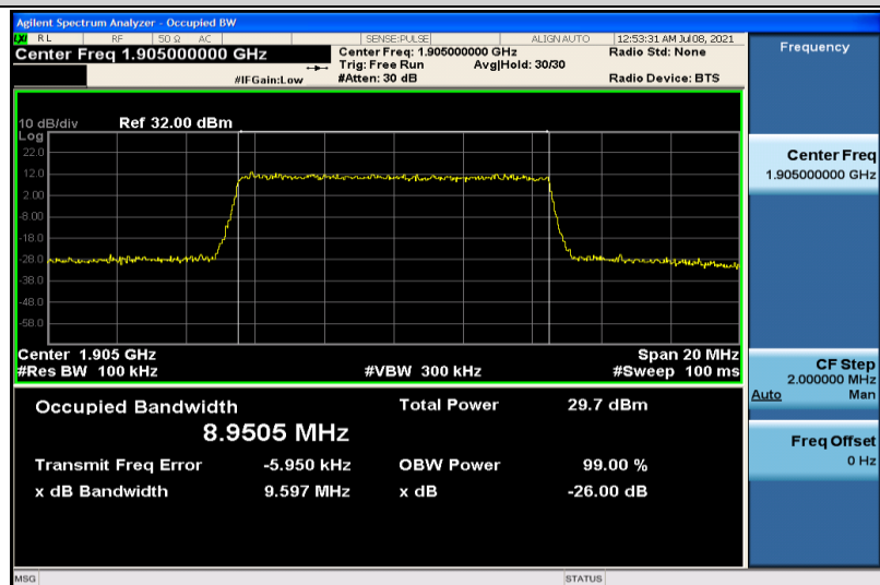
Band2-10MHz-QPSK-19150-50RB#0-8.9505
