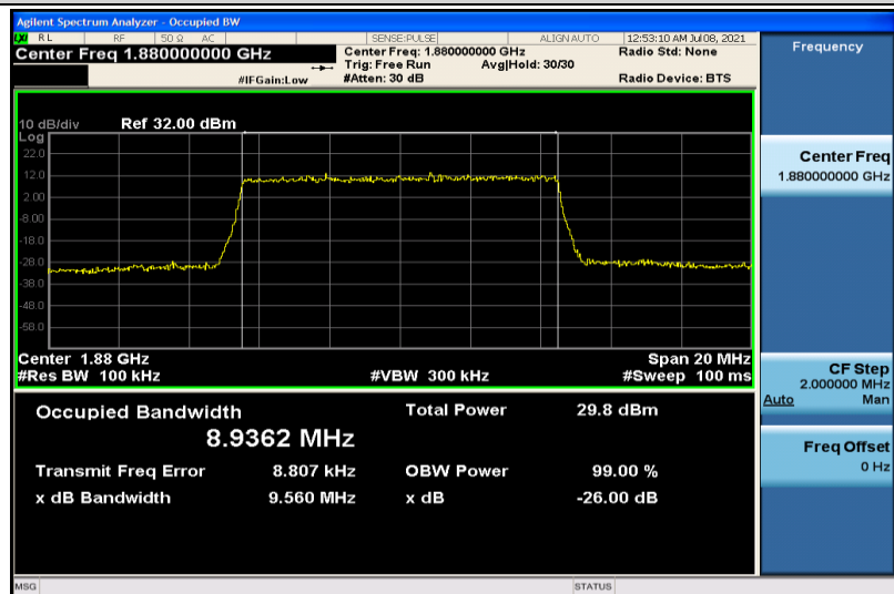
Band2-10MHz-QPSK-18900-50RB#0-8.9362
