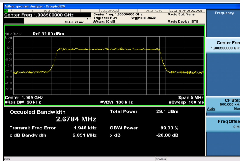
Band2-3MHz-QPSK-19185-15RB#0-2.6784
