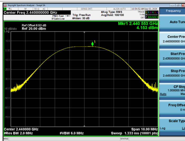
Peak Power NVNT BLE 2M 2440MHz Ant1
