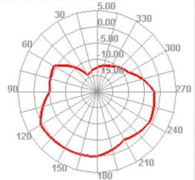
5600.000MHz E2
