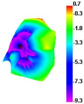
5500.000MHz E1
