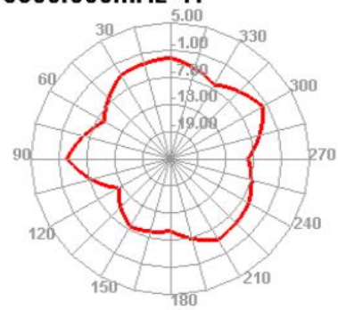
5800.000MHz H
