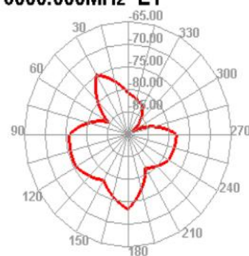
6000.000MHz E1
