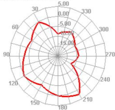
5600.000MHz E1
