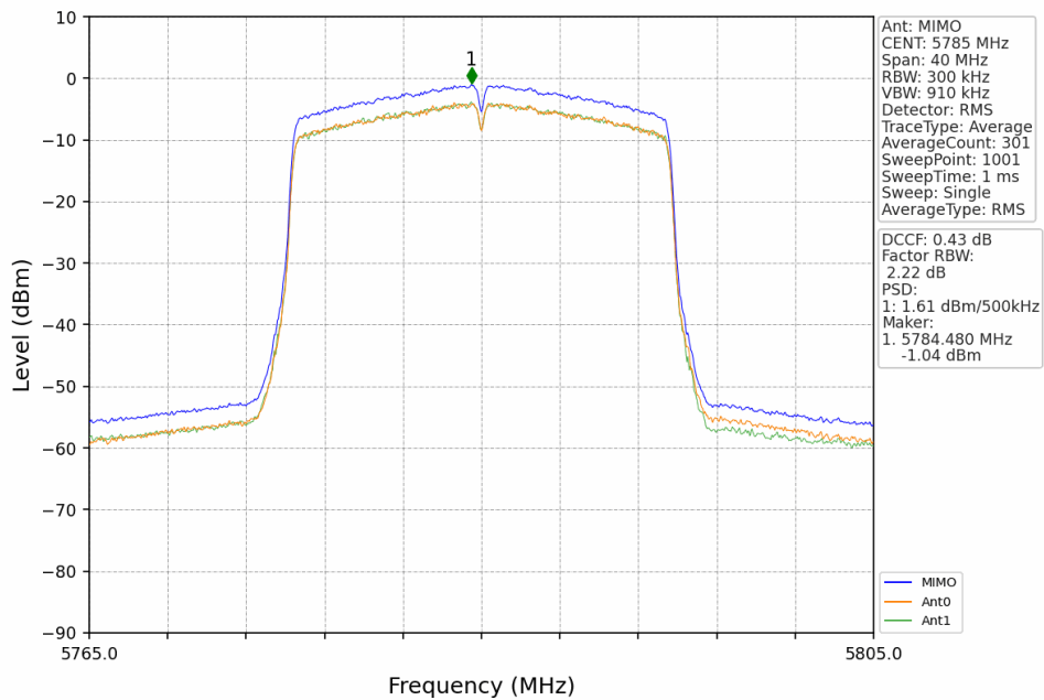
802.11ax(HEW20) MCH 5785MHz RU242 Left MIMO NTNV
