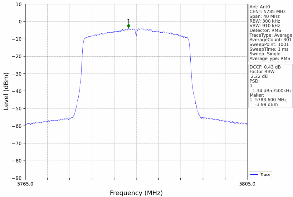
802.11ax(HEW20)_MCH_5785MHz_RU242_Left_Ant0_NTNV
