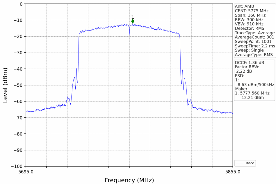
802.11ax(HEW80)_MCH_5775MHz_RU996_Left_Ant0_NTNV
