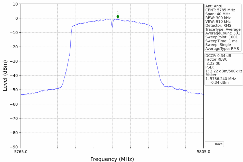
802.11n(HT20) MCH 5785MHz Ant0 NTN
