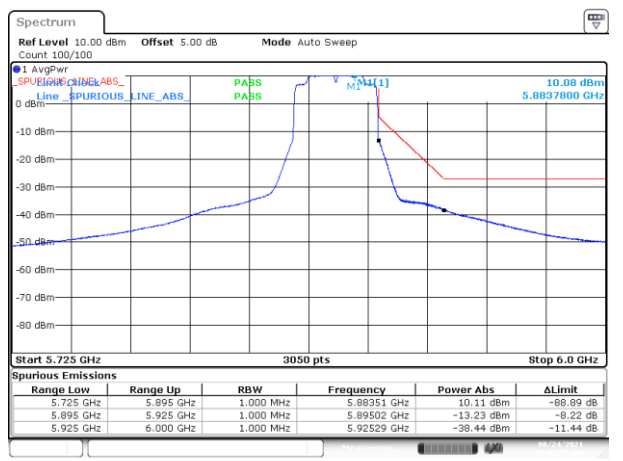
BE-NR-HIGH, SISO-A, 802.11ax40-HE0, Ch175
