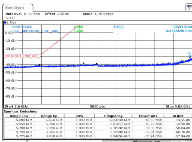
BE-NR-LOW, SISO-A, 802.11a20-6Mbps, Ch177
