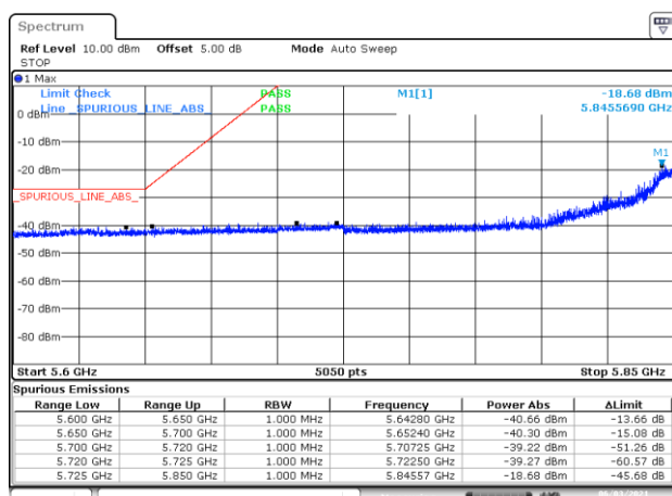
BE-NR-LOW, SISO-A, 802.11a20-6Mbps, Ch173
