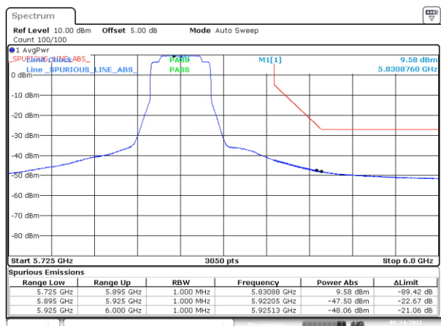
BE-NR-HIGH, SISO-A, 802.11ax40-HE0, Ch167
