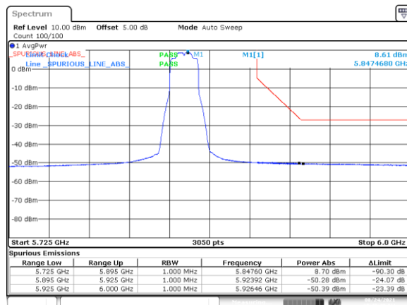
BE-NR-HIGH, MIMO-A, 802.11ax20-HE0, Ch169
