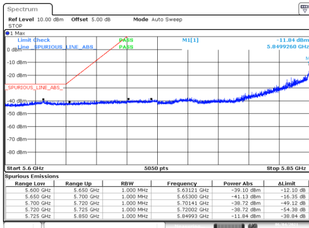
BE-NR-LOW, SISO-B, 802.11ax20-HE0, Ch173
