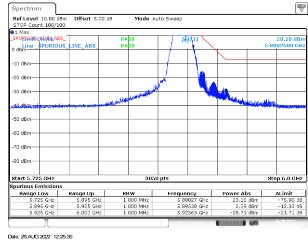
BE-NR-HIGH, SISO-A, 802.11a20-6Mbps, Ch177
