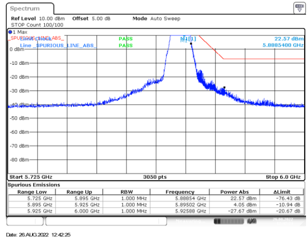
BE-NR-HIGH, SISO-A, 802.11n20-HT0, Ch177
