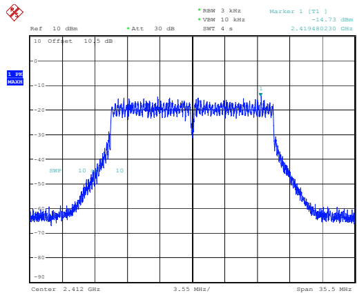
802.11n20_2412MHz
