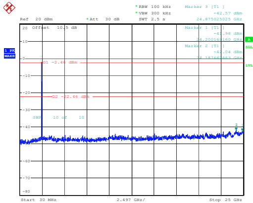
802.11b_2472MHz
