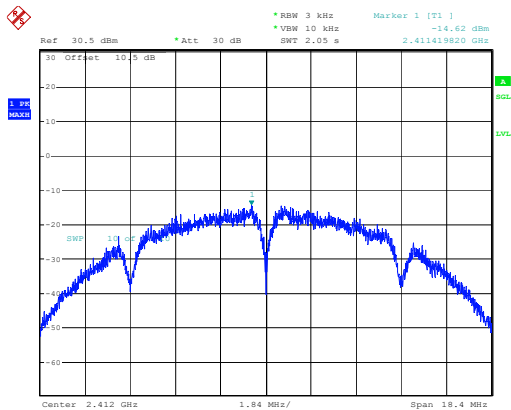
802.11b_2412MHz
