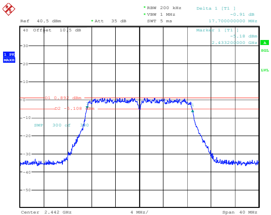
802.11n20_2442MHz
