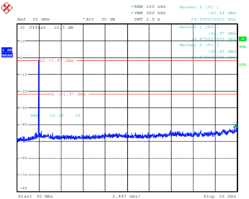
802.11b_2442MHz
