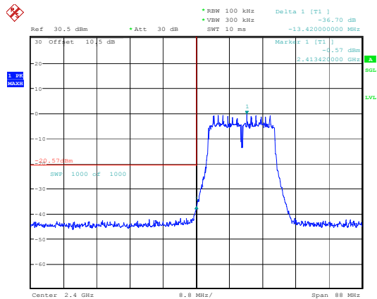
802.11n20_2412MHz
