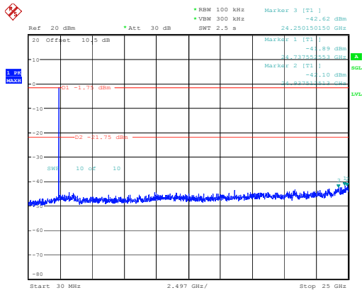
802.11b_2412MHz
