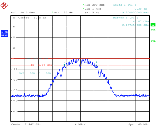
802.11b_2442MHz
