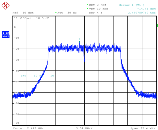
802.11n20_2442MHz
