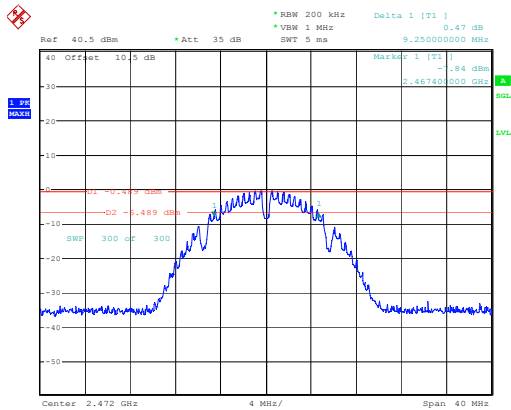
802.11b_2472MHz
