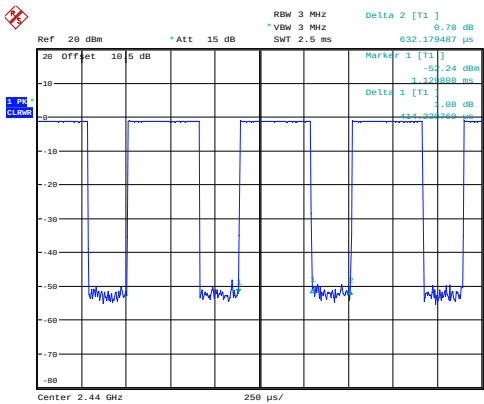
BLE 1Mbps Middle
