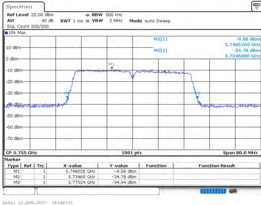
-26 dB BW NVNT 802.11ac40 5755MHz Ant 1
