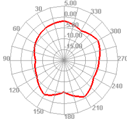
2350.000MHz E2
