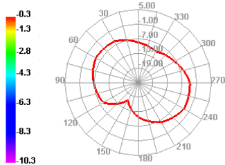
2350.000MHz E2
