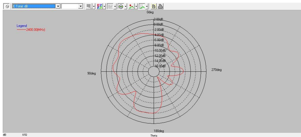
PHI90deg
