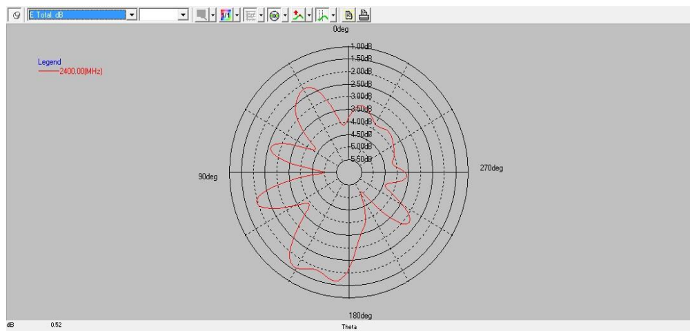
THETA90deg
