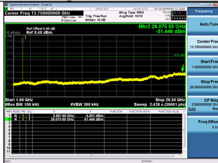
BLE 1M-Ant1-2402-1000~26500-PASS
