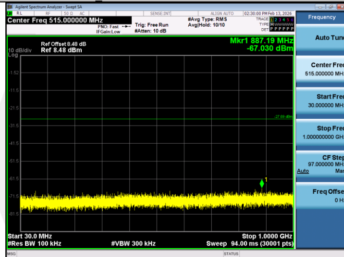
BLE_2M-Ant1-2402-30~1000-PASS
