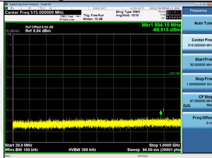
BLE_2M-Ant1-2480-30~1000-PASS
