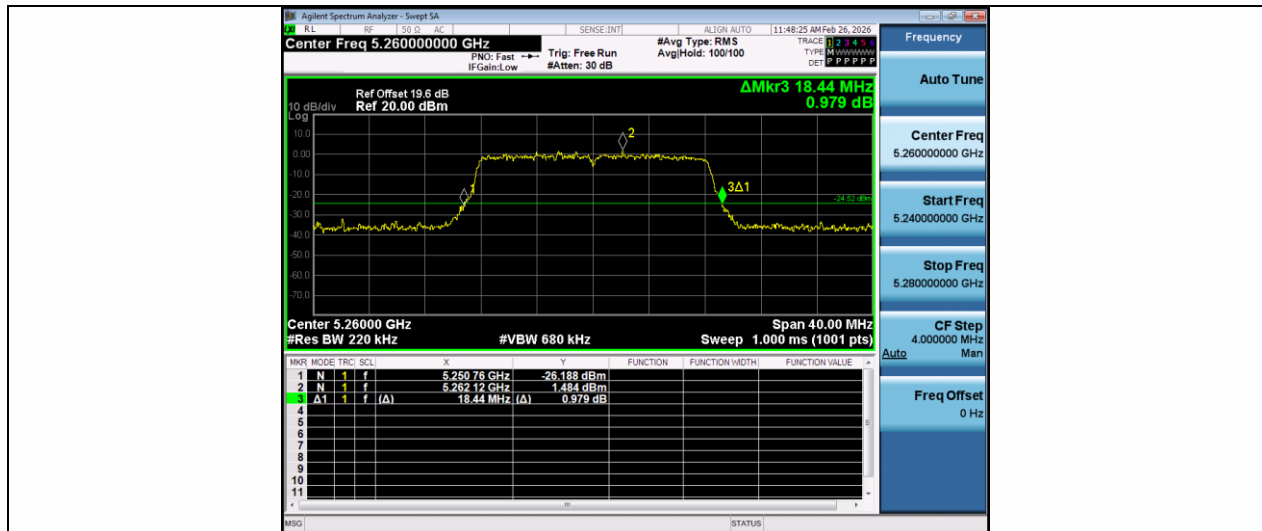
11A-Ant1-5260
