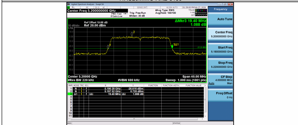
11AC20MIMO-Ant1-5200
