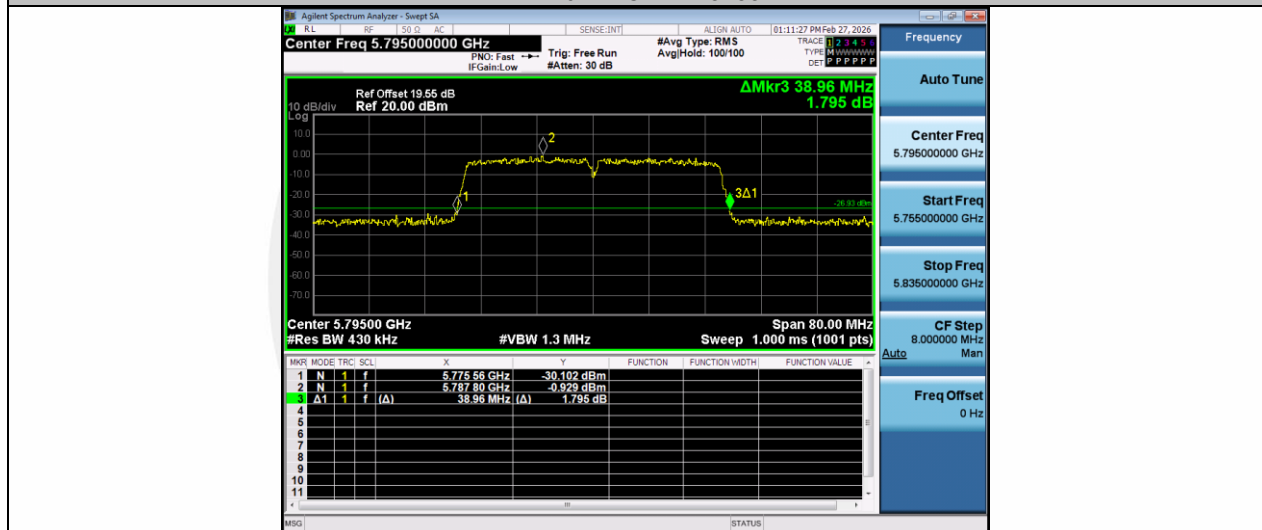
11N40MIMO-Ant1-5795
