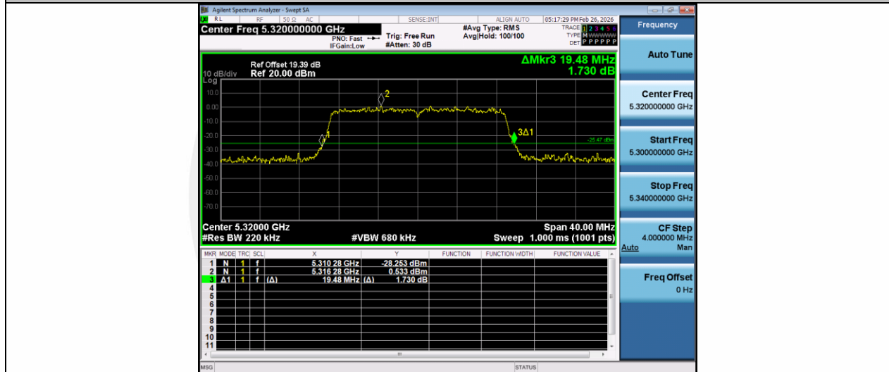
11N20MIMO-Ant1-5320
