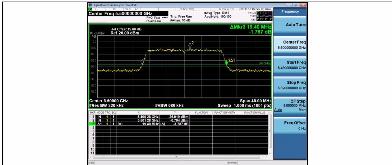
11N20MIMO-Ant1-5500
