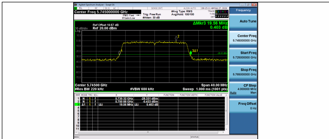
11N20MIMO-Ant1-5745
