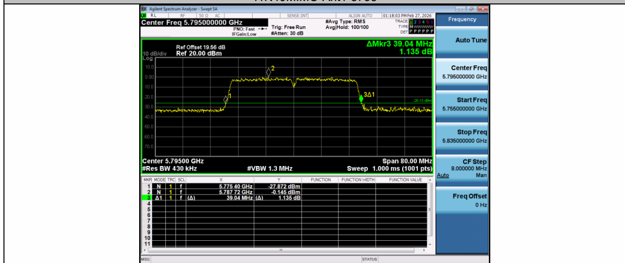
11N40MIMO-Ant2-5795
