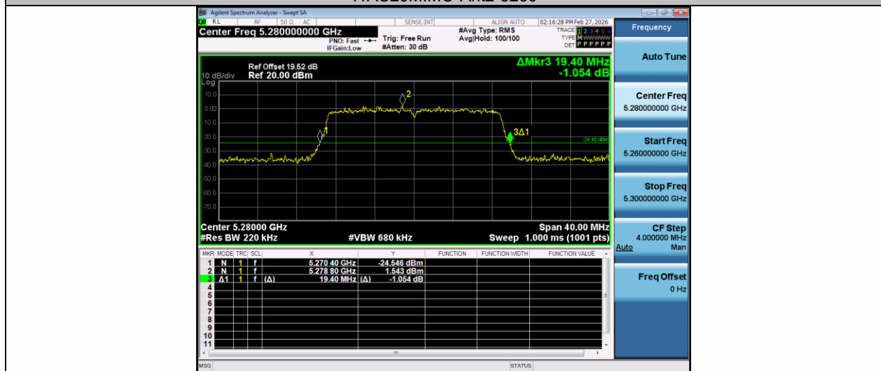
11AC20MIMO-Ant1-5280
