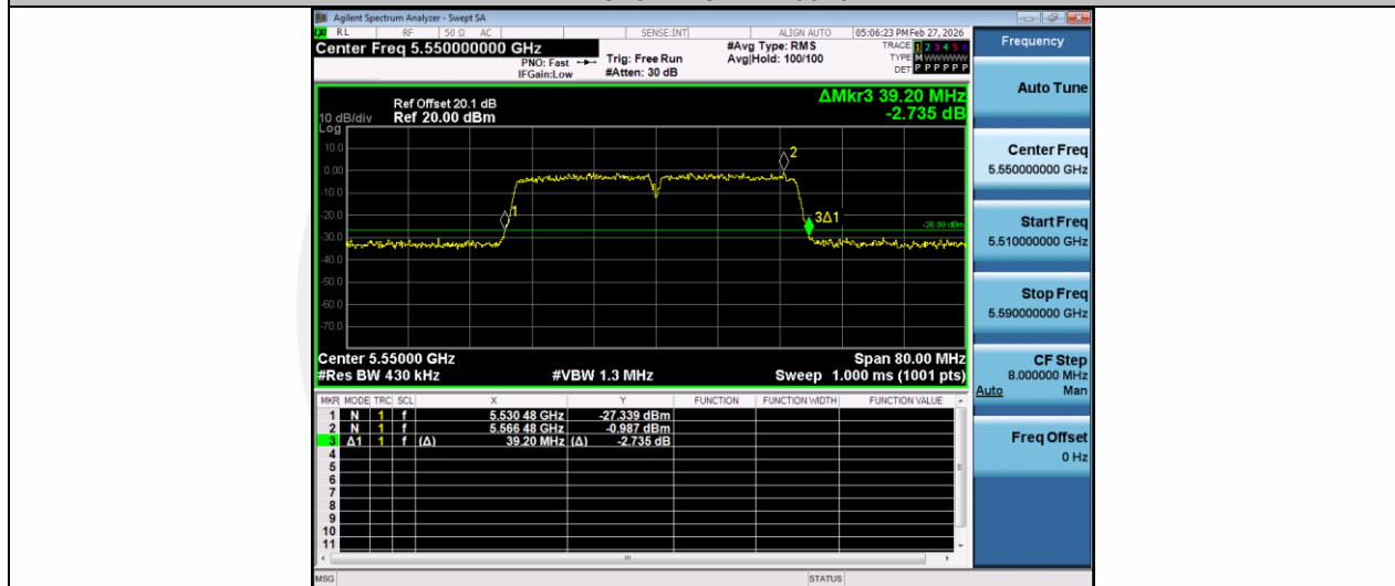
11AC40MIMO-Ant1-5550
