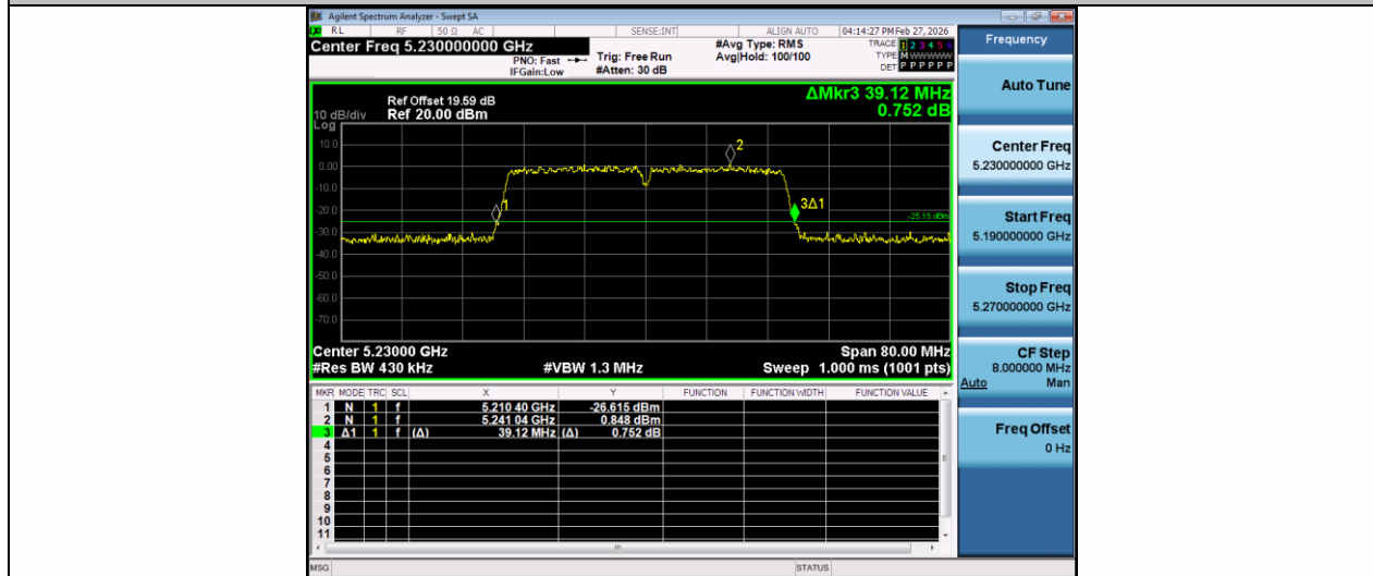
11AC40MIMO-Ant1-5230
