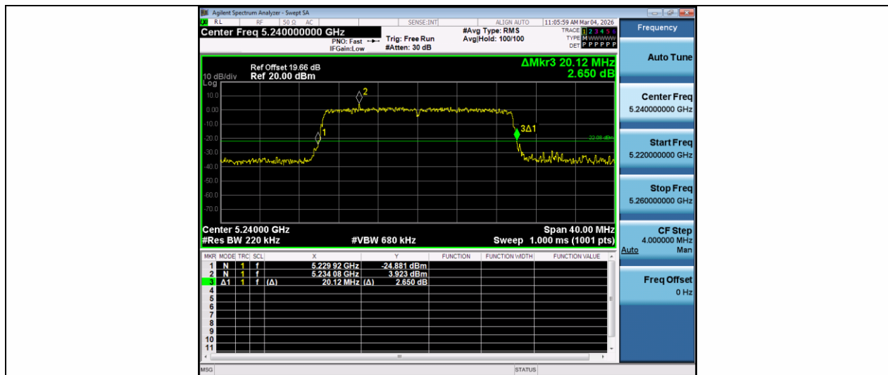
11AX20MIMO-Ant2-5240
