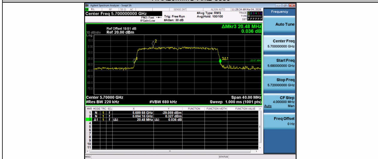
11AX20MIMO-Ant1-5700
