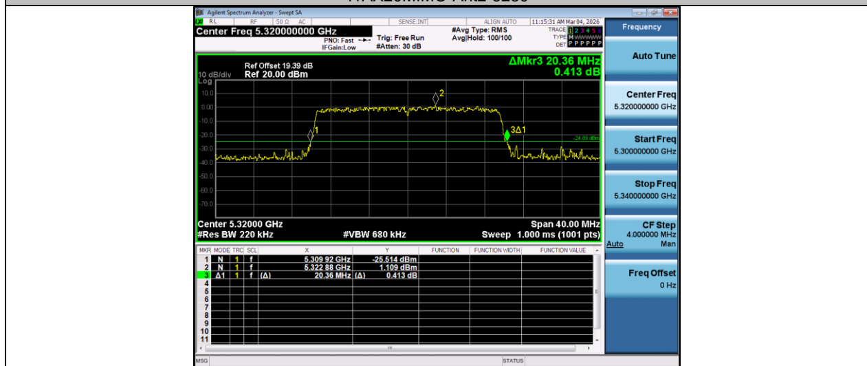
11AX20MIMO-Ant1-5320
