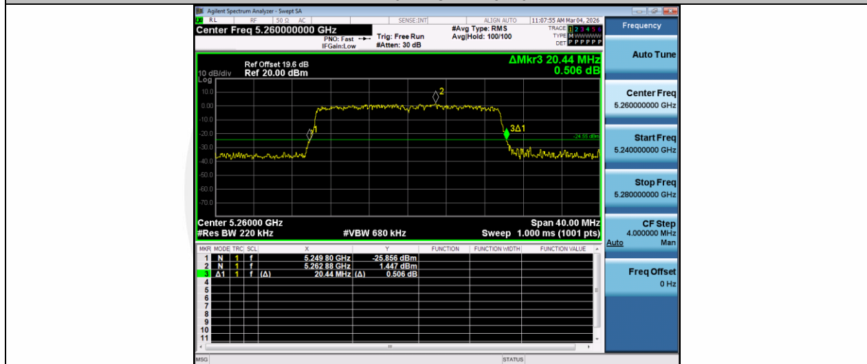
11AX20MIMO-Ant1-5260
