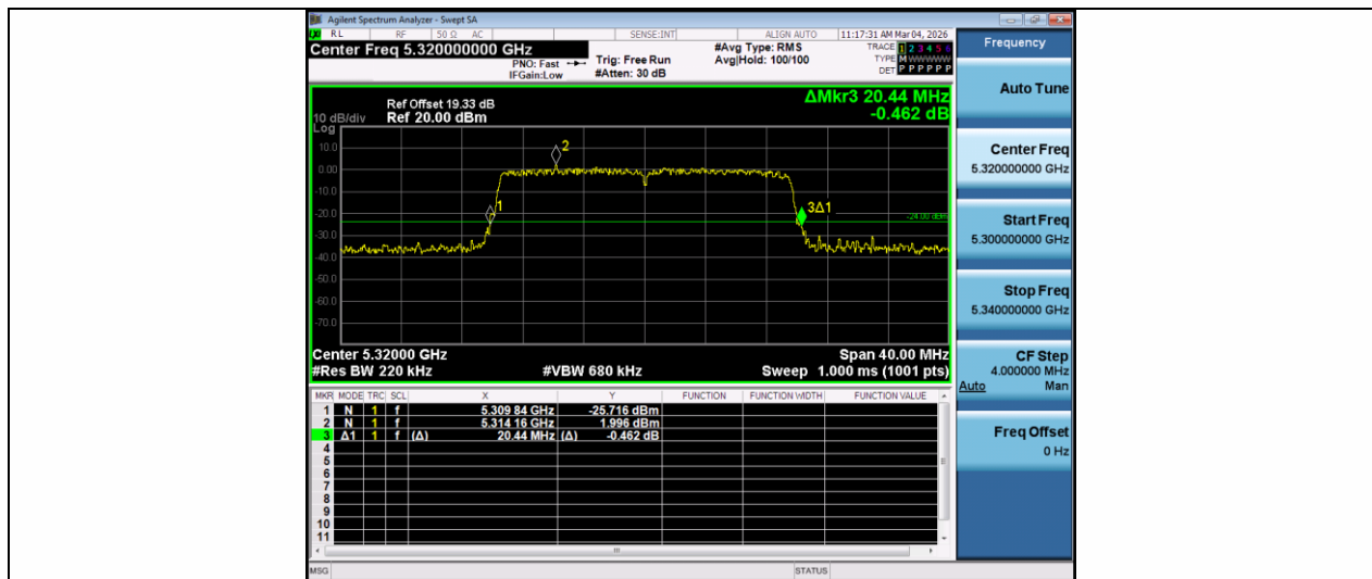
11AX20MIMO-Ant2-5320
