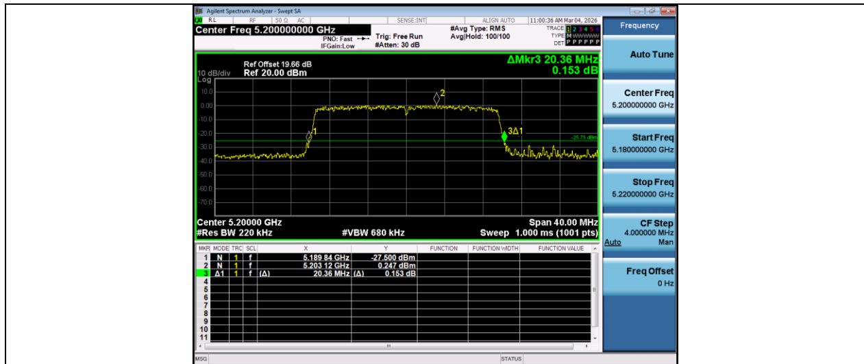
11AX20MIMO-Ant1-5200
