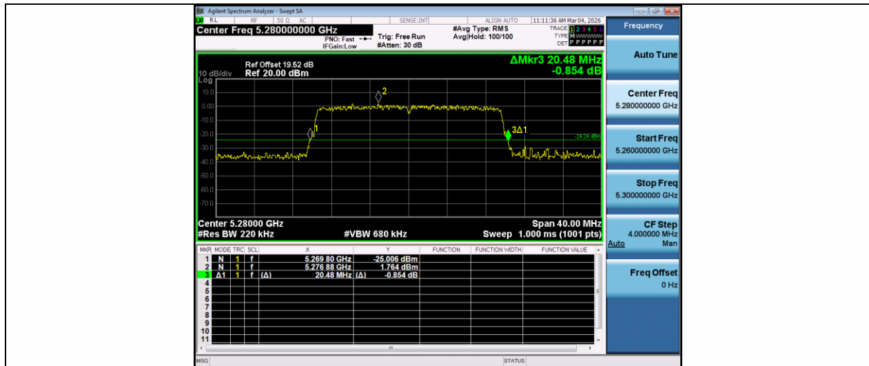
11AX20MIMO-Ant1-5280
