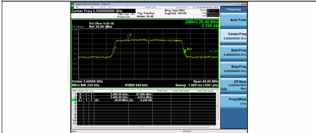
11AX20MIMO-Ant1-5500
