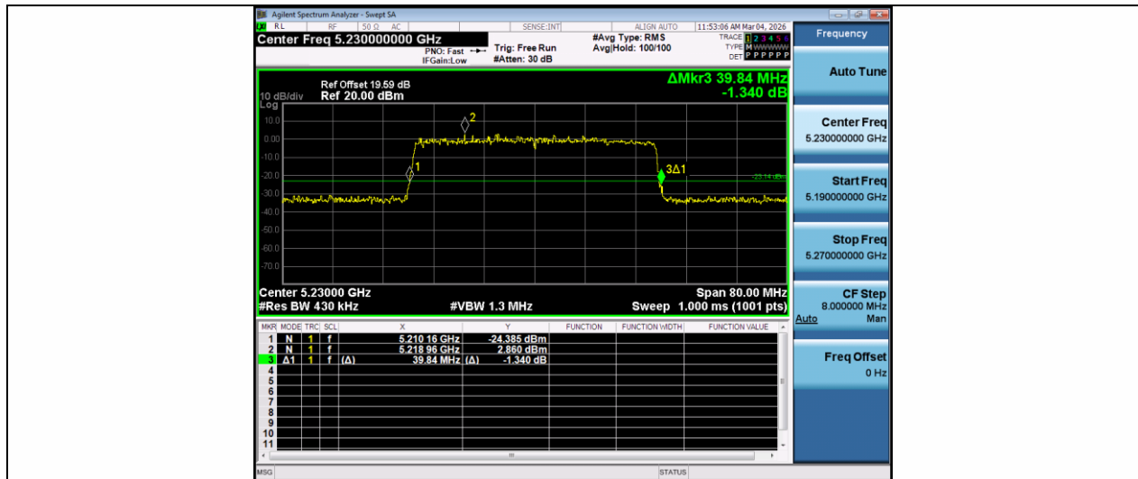
11AX40MIMO-Ant1-5230
