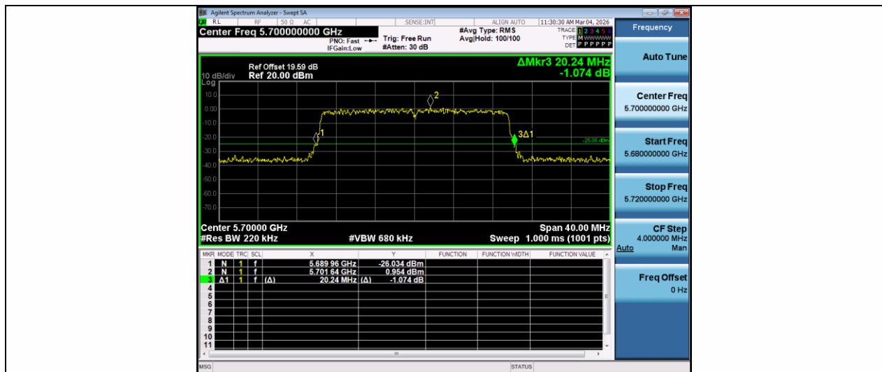
11AX20MIMO-Ant2-5700
