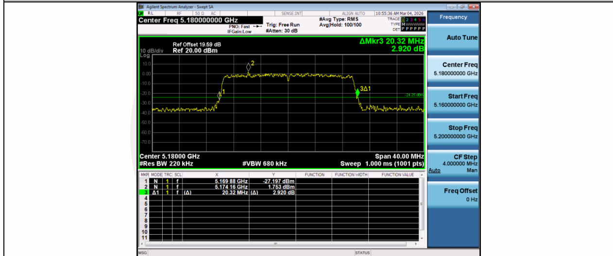
11AX20MIMO-Ant1-5180
