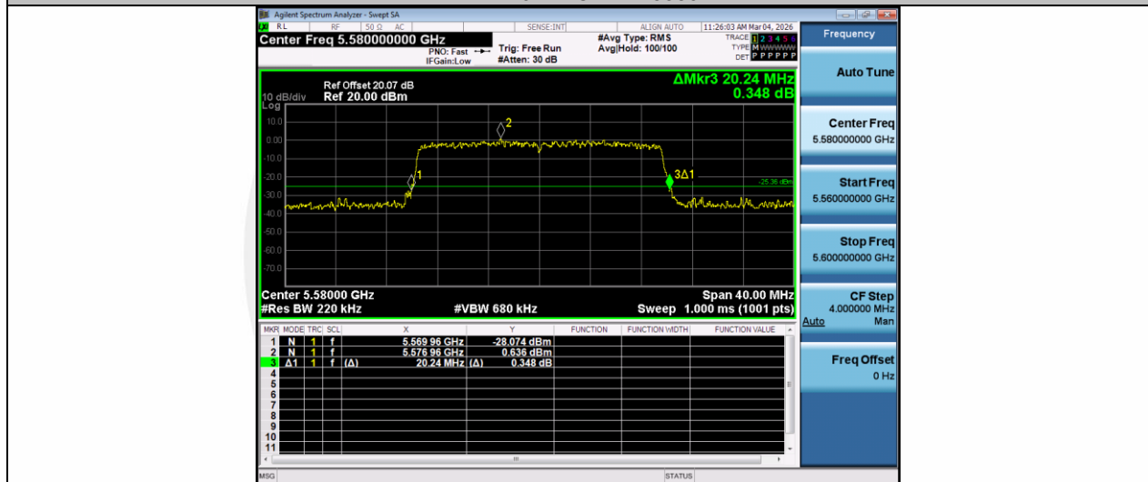
11AX20MIMO-Ant2-5580
