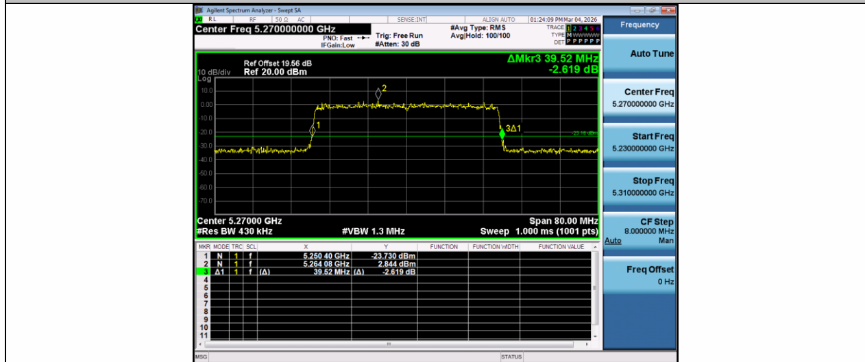
11AX40MIMO-Ant1-5270
