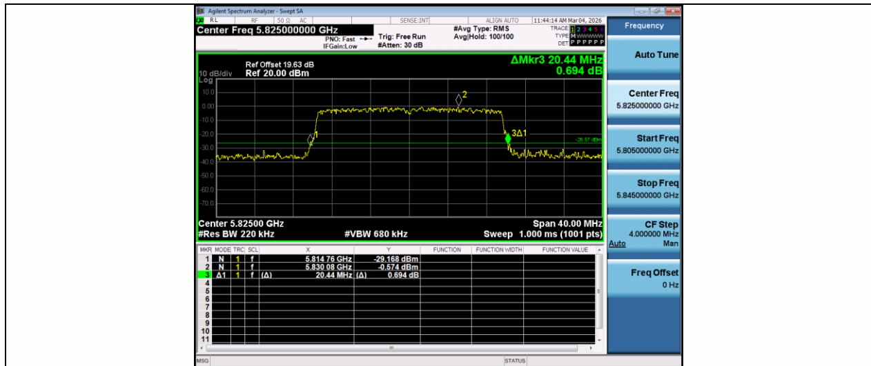
11AX20MIMO-Ant2-5825
