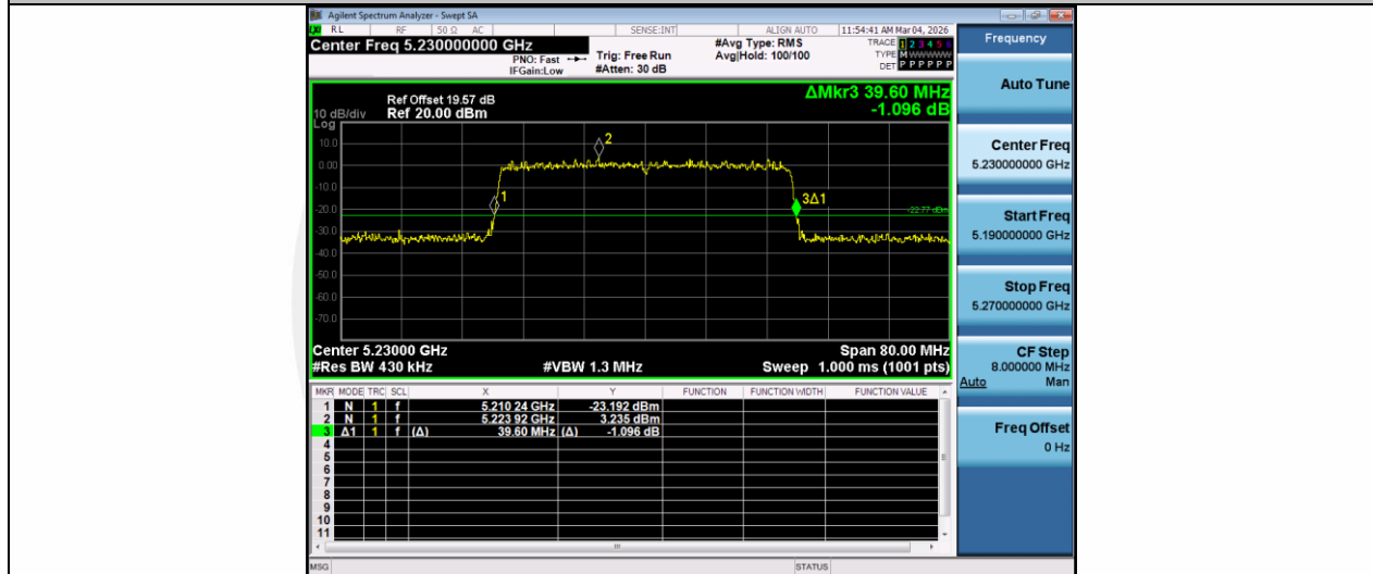
11AX40MIMO-Ant2-5230
