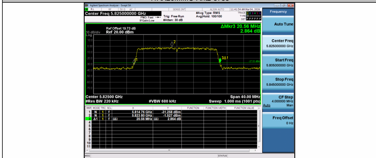
11AX20MIMO-Ant1-5825
