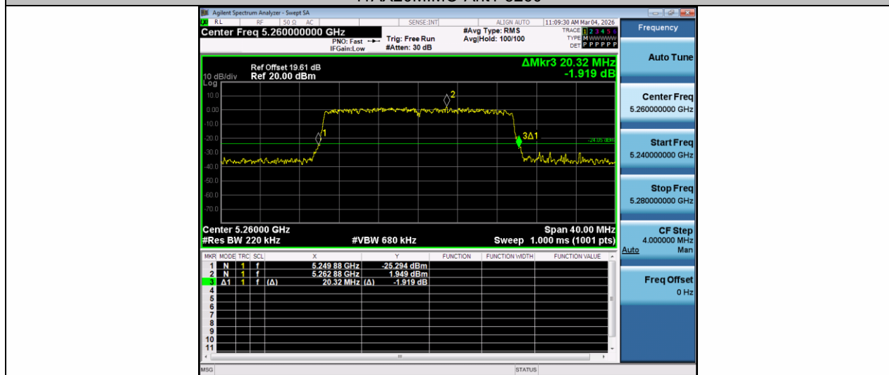
11AX20MIMO-Ant2-5260
