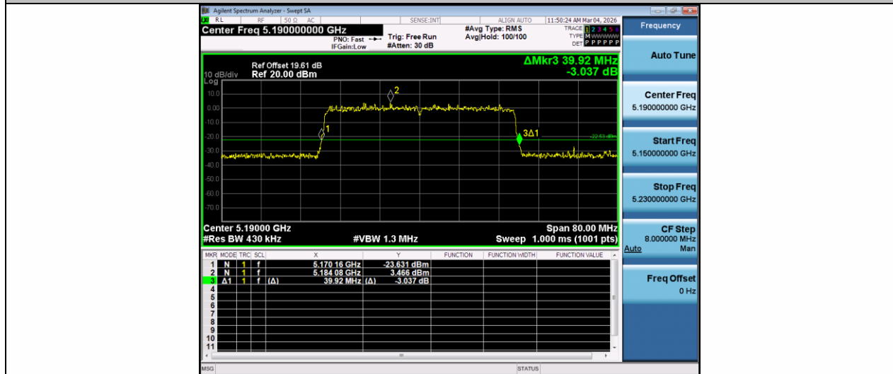
11AX40MIMO-Ant2-5190
