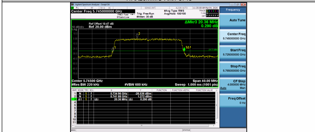
11AX20MIMO-Ant2-5745
