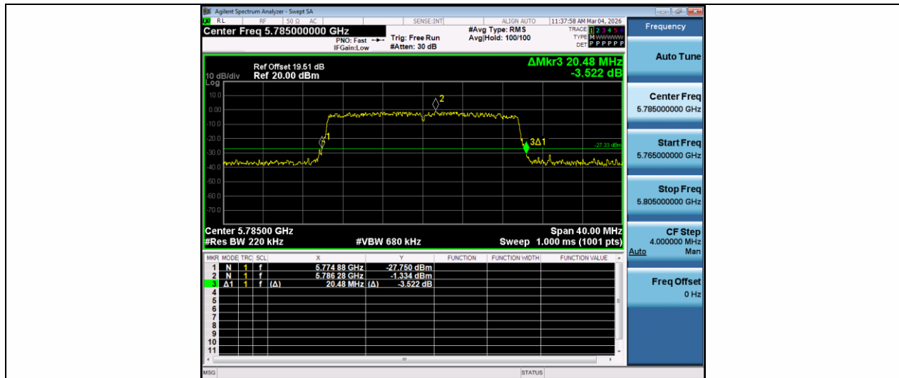
11AX20MIMO-Ant1-5785
