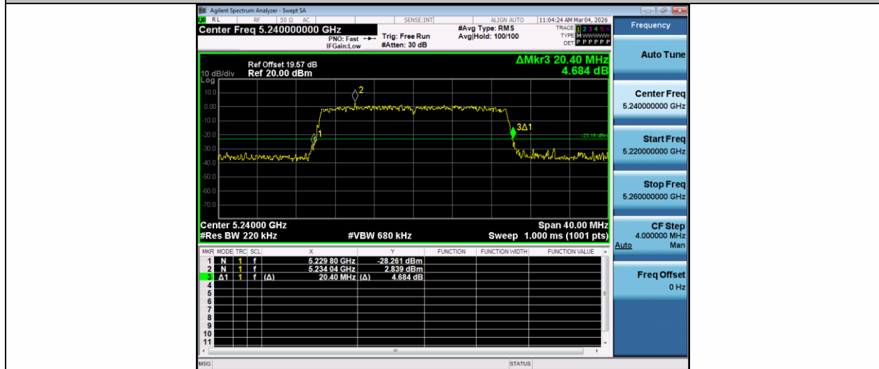
11AX20MIMO-Ant1-5240
