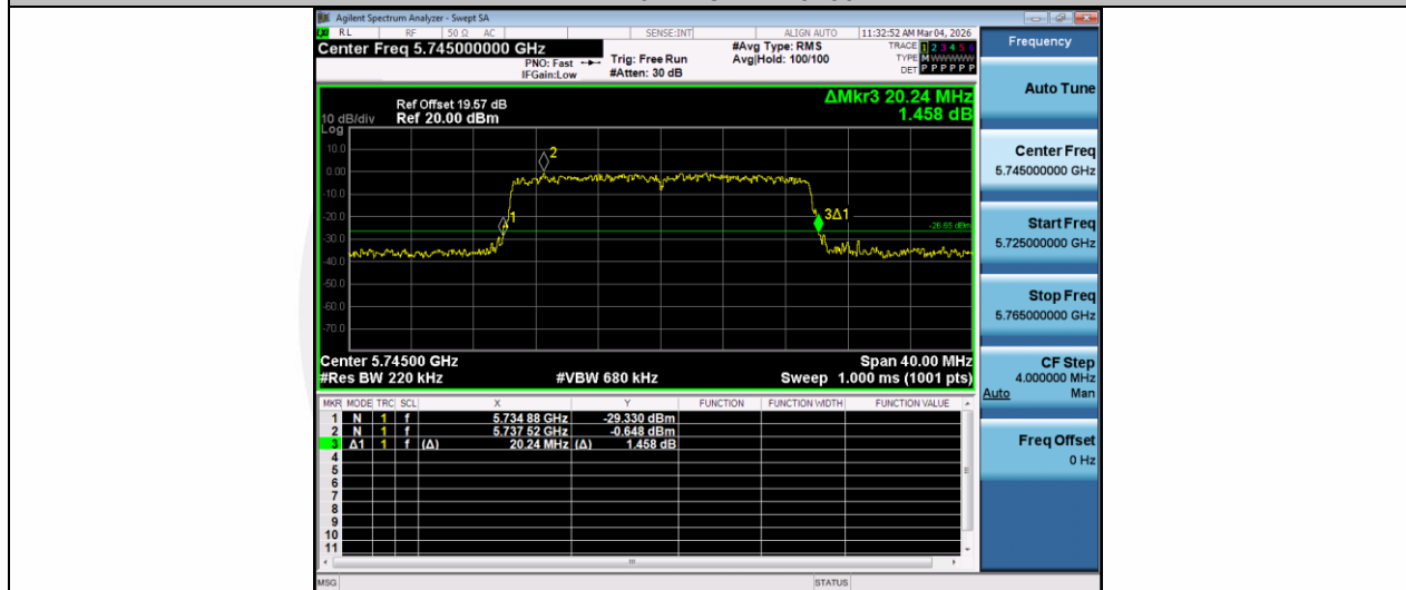
11AX20MIMO-Ant1-5745
