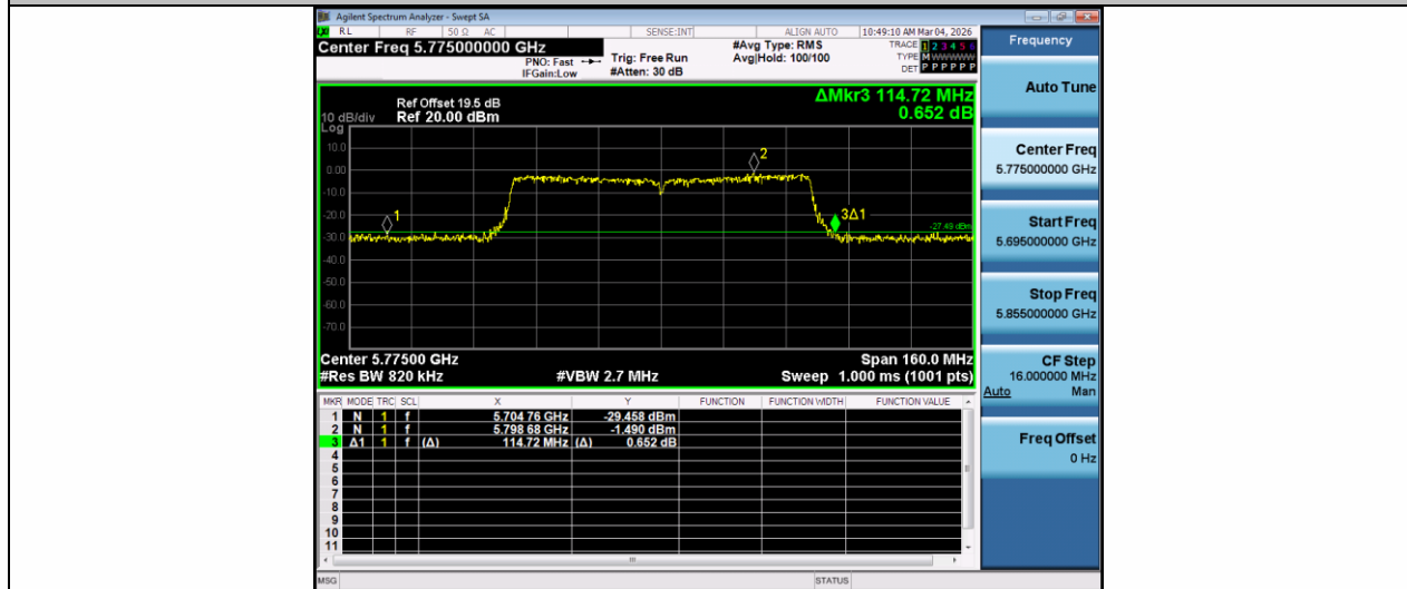
11AC80MIMO-Ant1-5775
