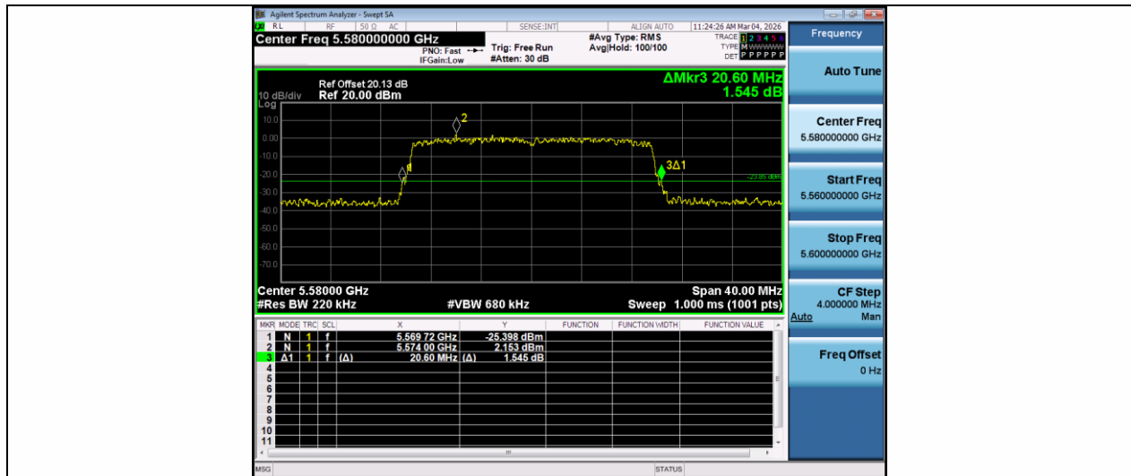
11AX20MIMO-Ant1-5580
