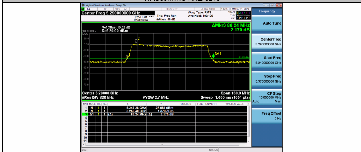
11AC80MIMO-Ant1-5290
