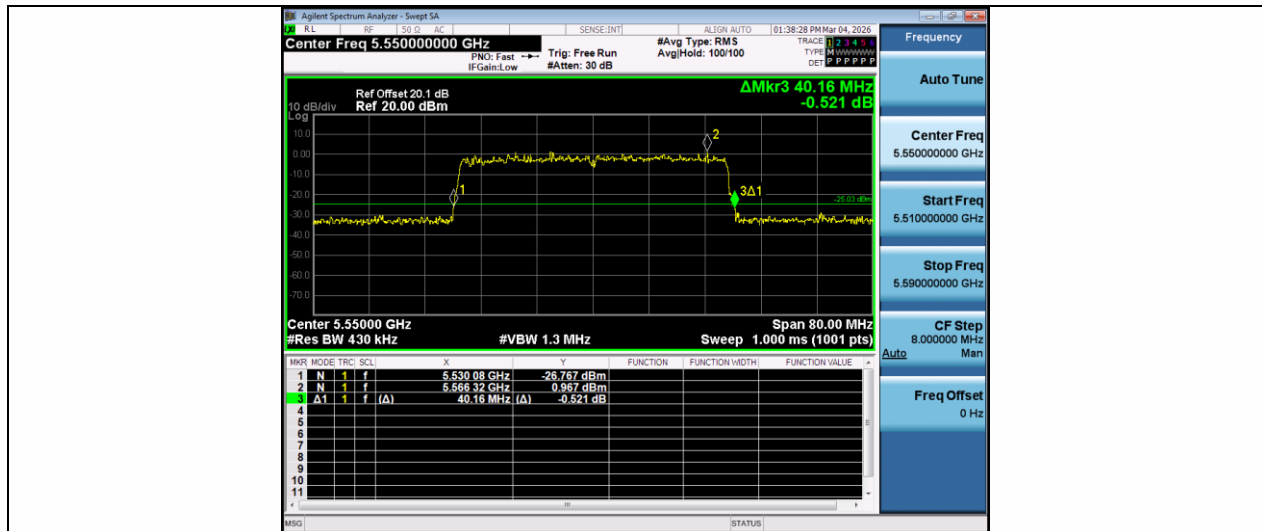
11AX40MIMO-Ant2-5550
