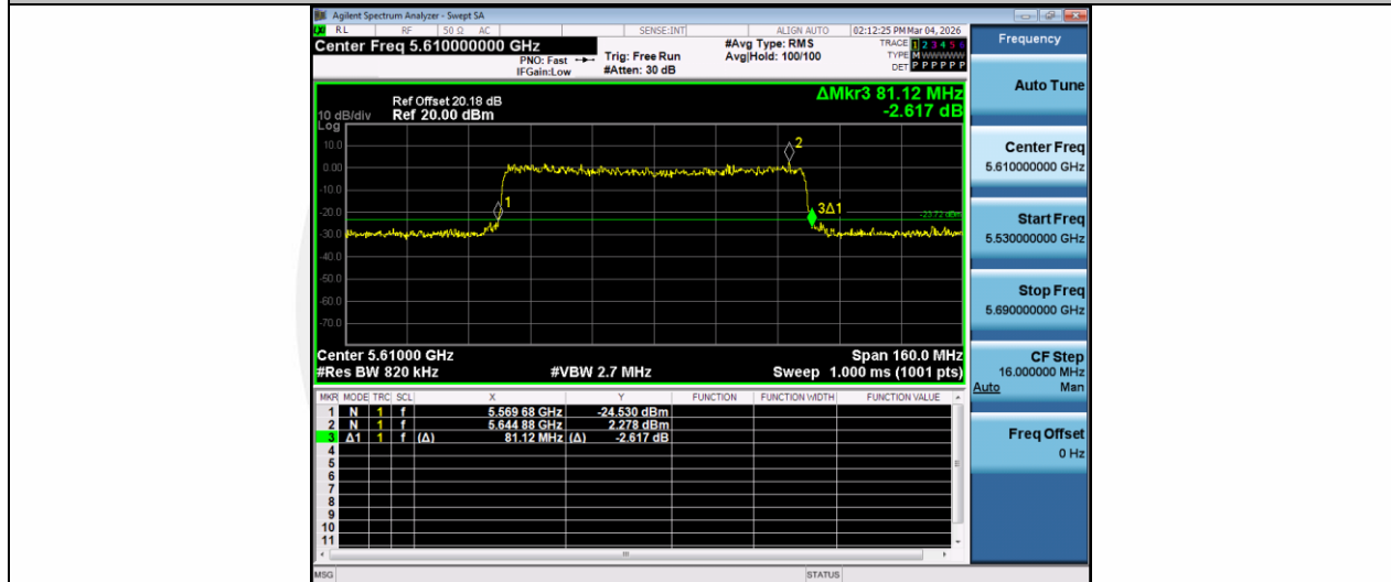
11AX80MIMO-Ant1-5610
