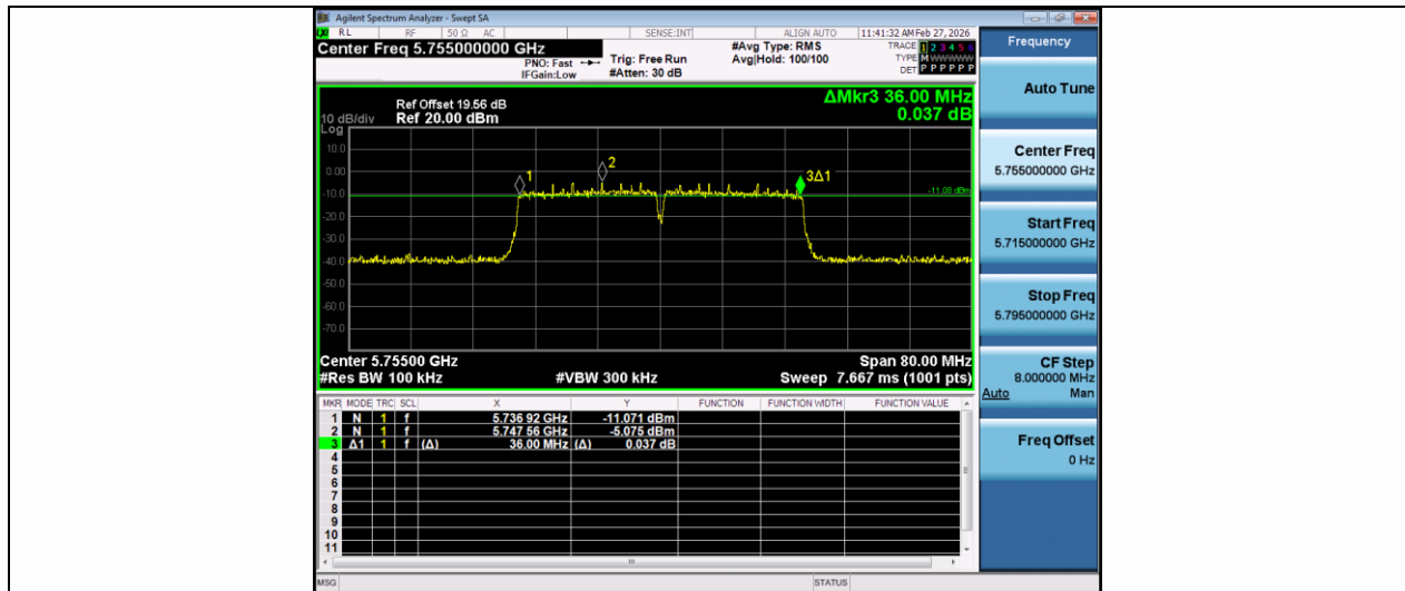
11N40MIMO-Ant1-5755-PASS
