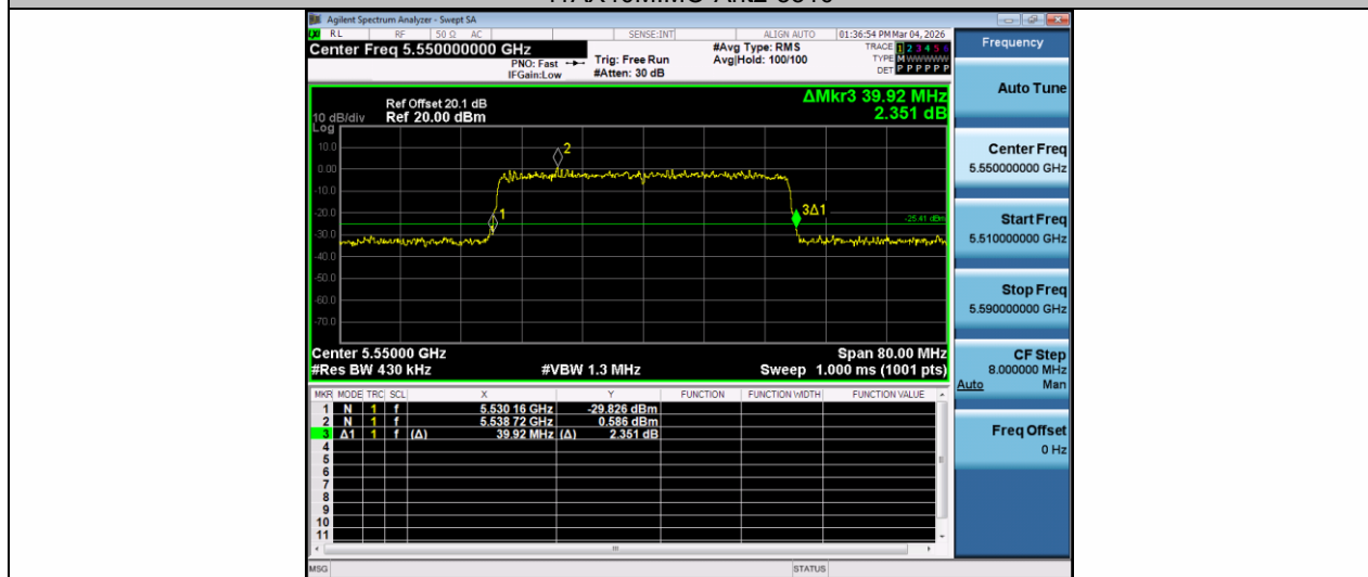
11AX40MIMO-Ant1-5550
