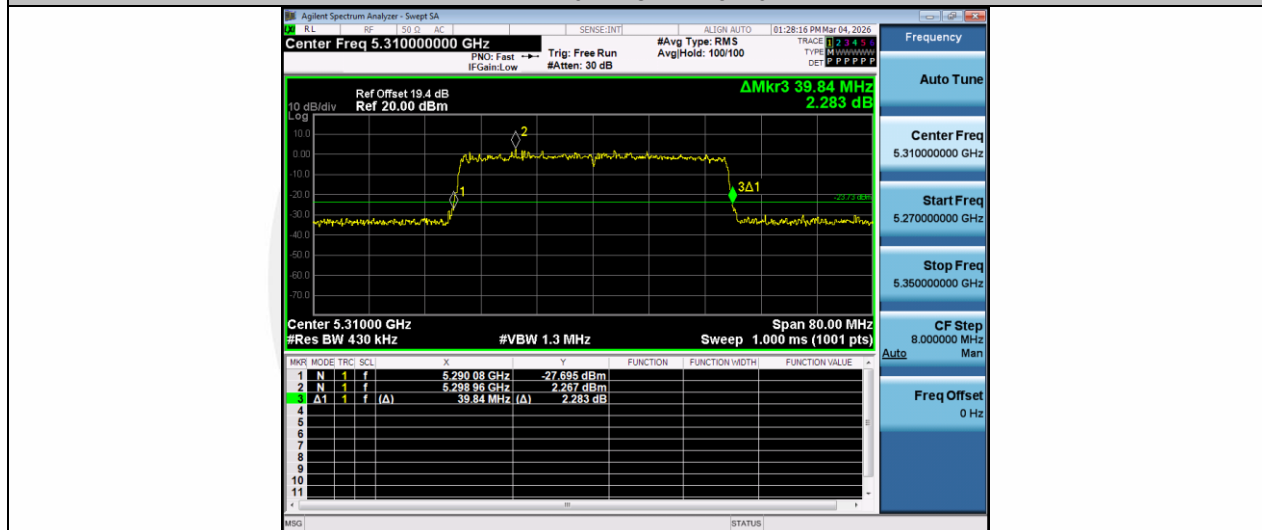
11AX40MIMO-Ant1-5310
