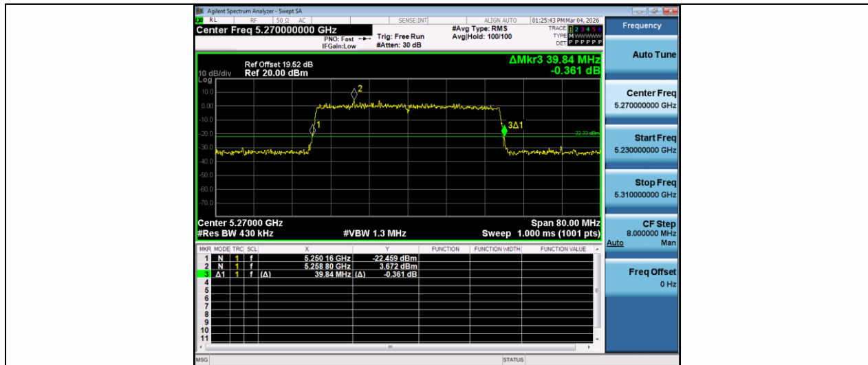
11AX40MIMO-Ant2-5270
