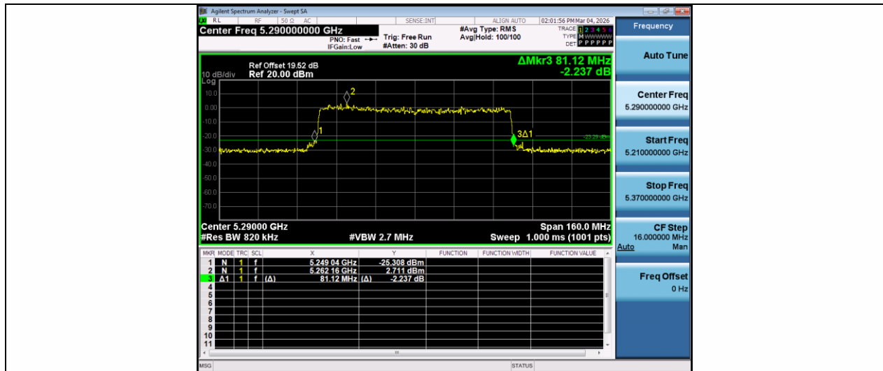
11AX80MIMO-Ant1-5290
