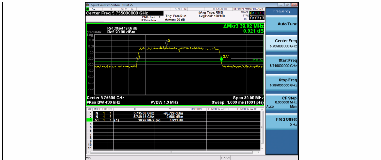
11AX40MIMO-Ant1-5755
