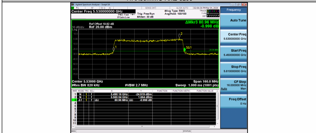
11AX80MIMO-Ant1-5530
