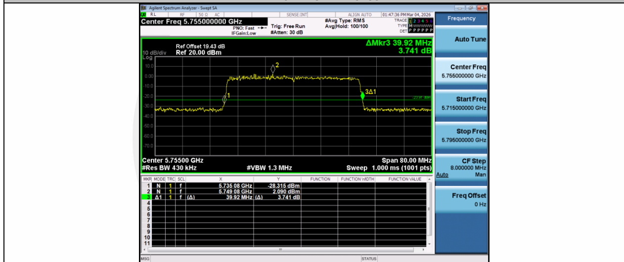
11AX40MIMO-Ant2-5755
