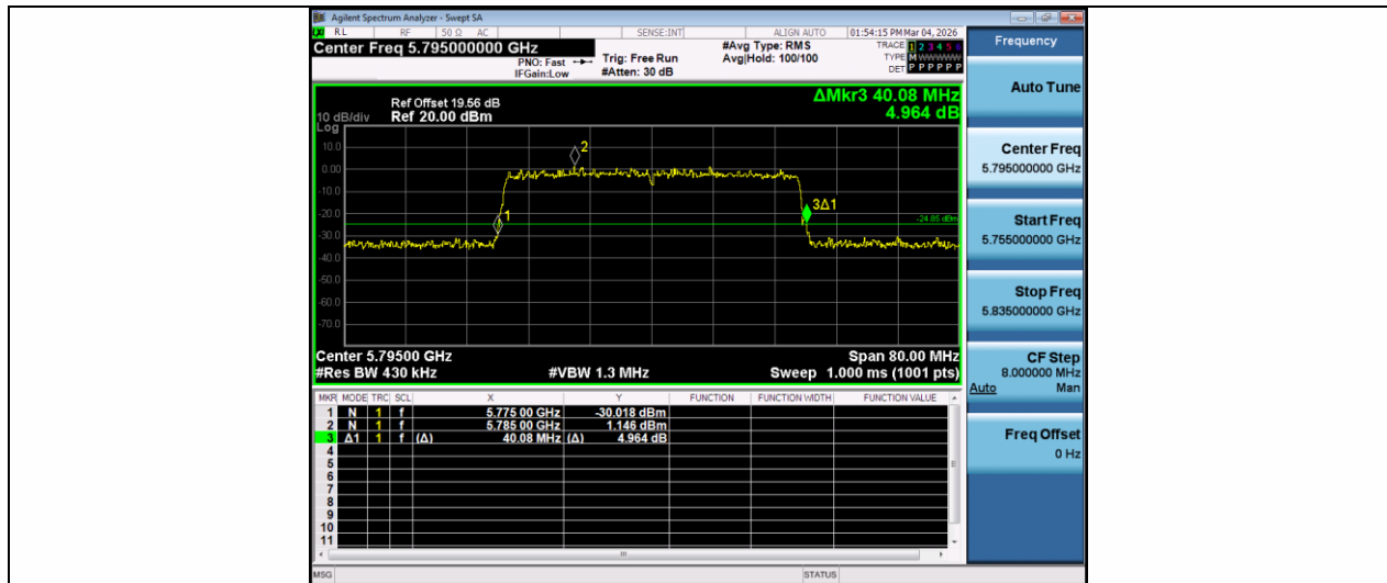
11AX40MIMO-Ant2-5795
