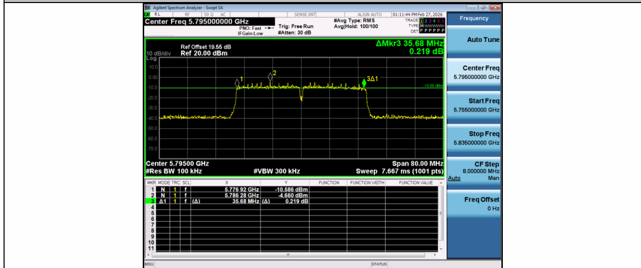
11N40MIMO-Ant1-5795-PASS
