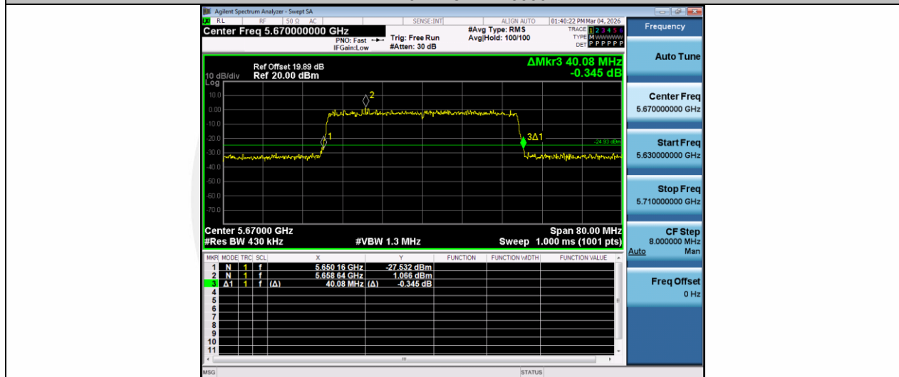
11AX40MIMO-Ant1-5670
