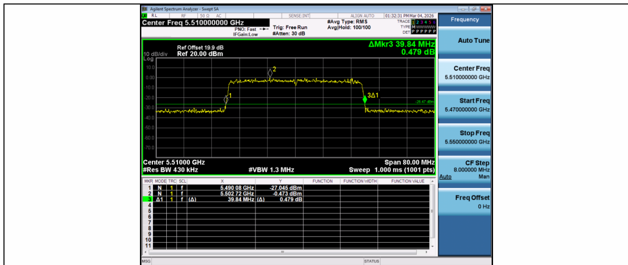
11AX40MIMO-Ant1-5510
