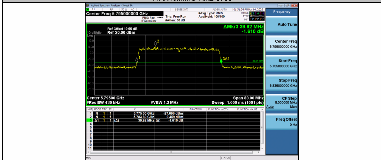
11AX40MIMO-Ant1-5795
