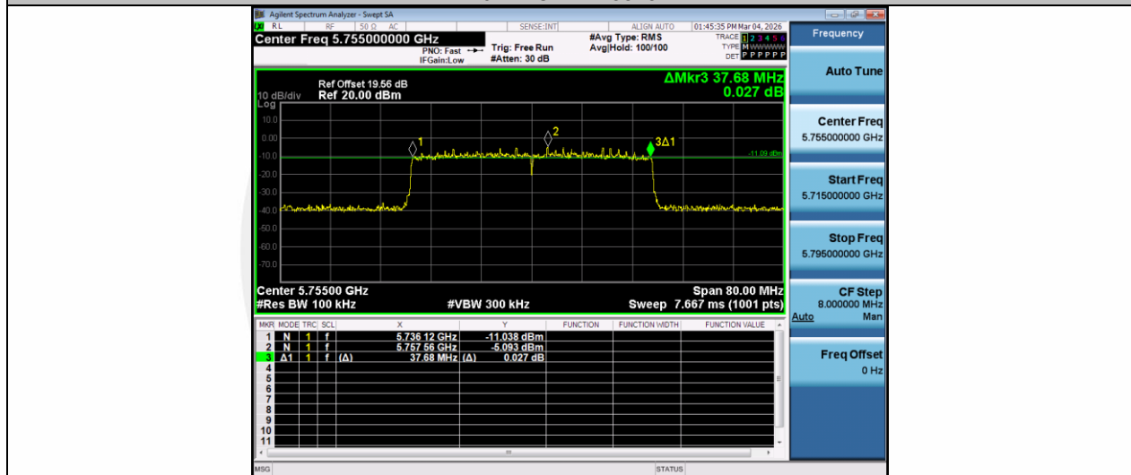
11AX40MIMO-Ant1-5755-PASS
