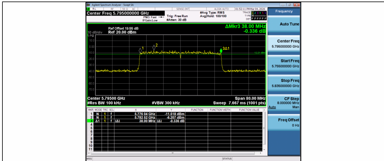
11AX40MIMO-Ant1-5795-PASS
