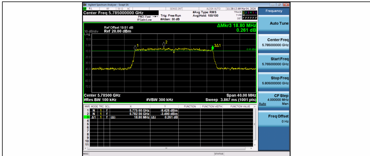
11AX20MIMO-Ant1-5785-PASS
