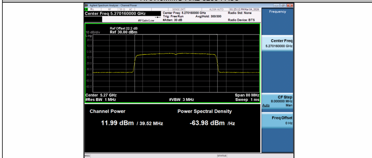
11AX40MIMO-Ant1-5270-PASS
