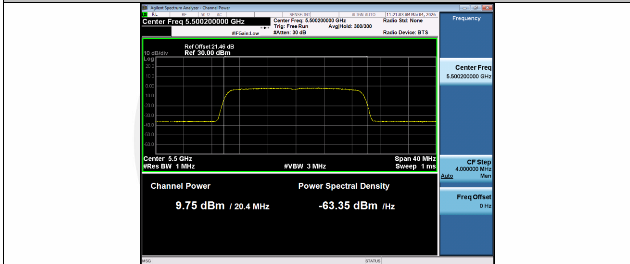
11AX20MIMO-Ant1-5500-PASS
