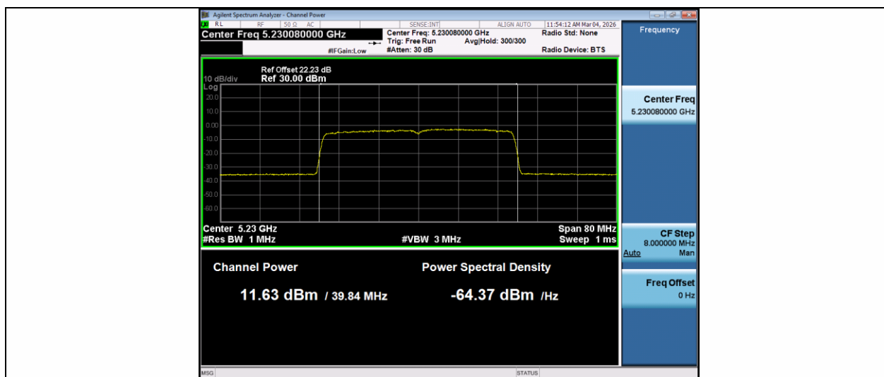
11AX40MIMO-Ant1-5230-PASS
