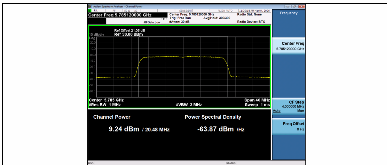
11AX20MIMO-Ant1-5785-PASS
