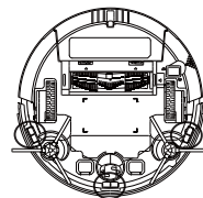
③ 3 sensori anticaduta in basso
