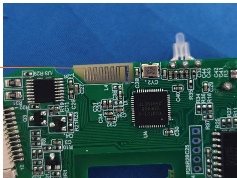
BLE ANT
