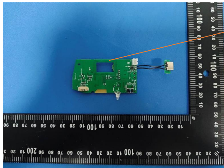
NFC ANT
