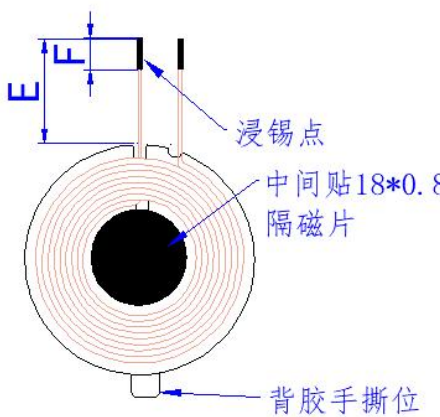
图三、线圈与磁片组合
