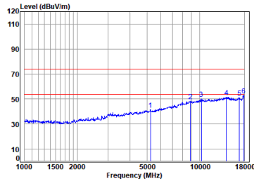
2.4G_SRD_2M_TX_CH_39_Horizontal
