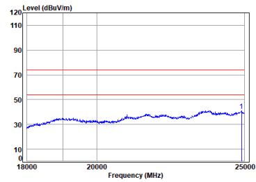
2.4G_SRD_TX_CH_39_Vertical
