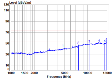
2.4G_SRD_TX_CH_39_Vertical
