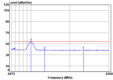
2.4G_SRD_1M_TX_CH_39_Horizontal-AVG
