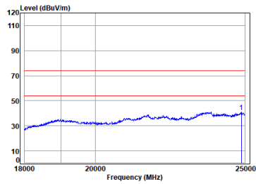
2.4G_SRD_TX_CH_39_Horizontal
