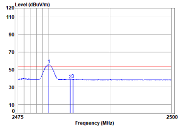
2.4G_SRD_1M_TX_CH_39_Vertical-AVG
