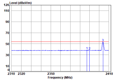
2.4G_SRD_2M_TX_CH_01_Vertical-AVG
