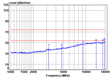
2.4G_SRD_2M_TX_CH_39_Vertical
