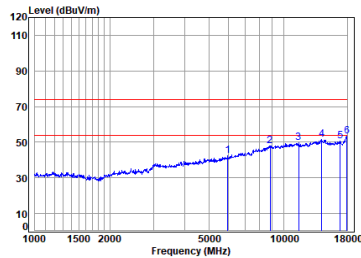
2.4G_SRD_TX_CH_19_Horizontal
