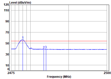
2.4G_SRD_2M_TX_CH_38_Horizontal-AVG
