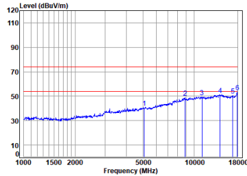
2.4G_SRD_2M_TX_CH_19_Horizontal
