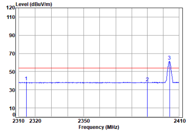
2.4G_SRD_2M_TX_CH_01_Horizontal-AVG
