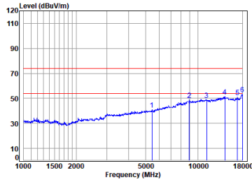
2.4G_SRD_TX_CH_39_Horizontal
