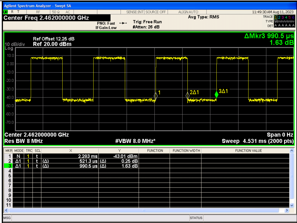
IEEE 802.11n_20MHz_Channel 11
