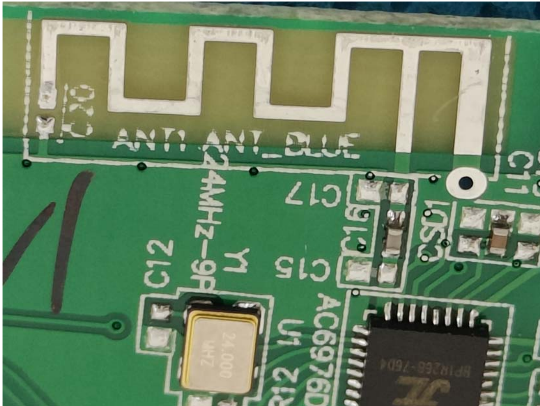
Model: K1 (Pink) _ Antenna
