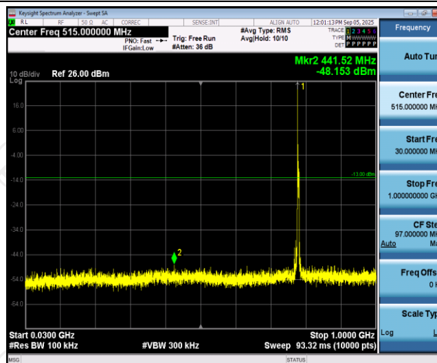
Band13-5MHz-QPSK-23255-1RB#0-Range1:30~1000MHz
