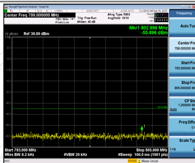
Band13-5MHz-QPSK-23230-1RB#0-Range4:793~805MHz
