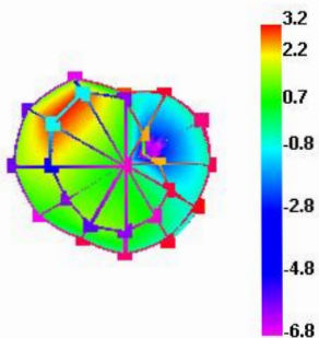
2040.000MHz
