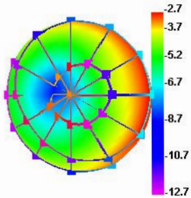
850.000MHz
