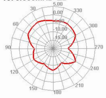
1870.000MHz E2
