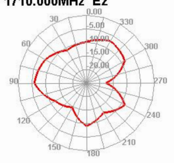
1710.000MHz E2
