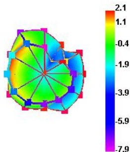
2450.000MHz
