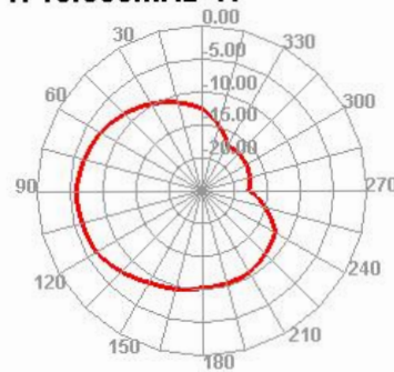
1710.000MHz H
