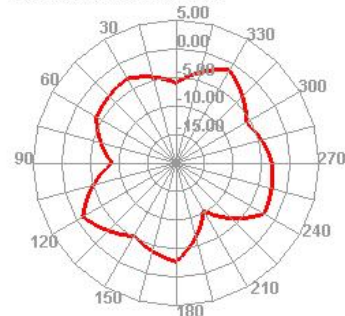
1575.000MHz E2
