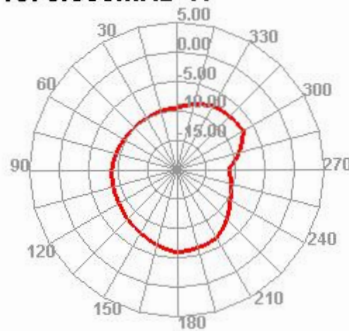
1870.000MHz H
