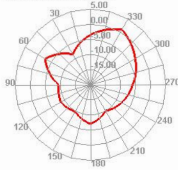
1870.000MHz E1
