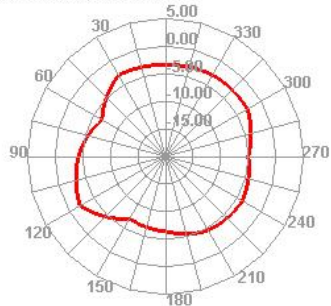
2450.000MHz H
