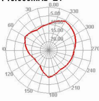
1710.000MHz E1
