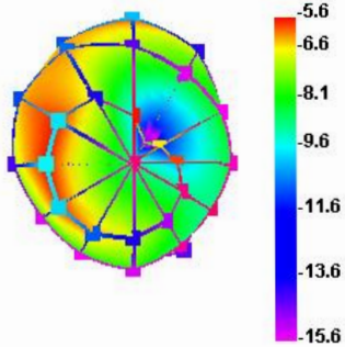
1710.000MHz
