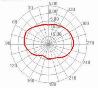
850.000MHz E2
