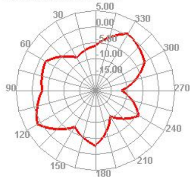
1575.000MHz E1
