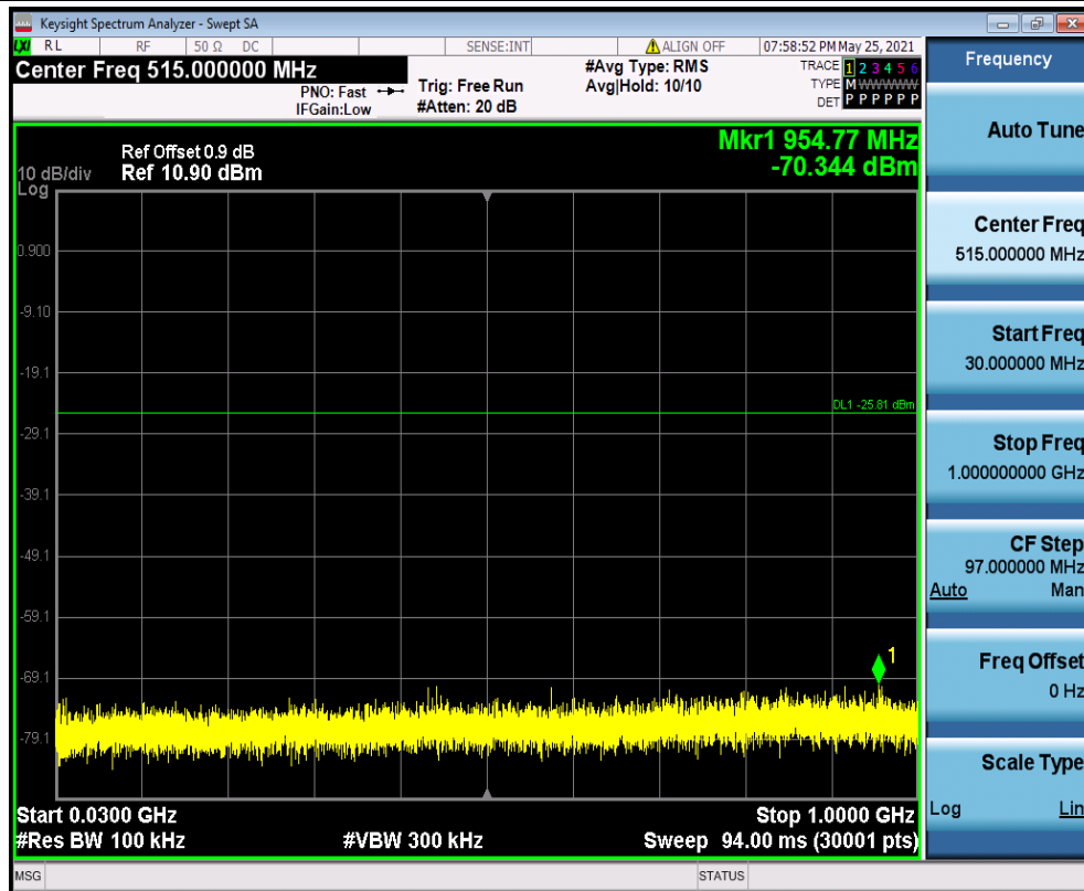
DH5_Ant1_2480_30-1000
