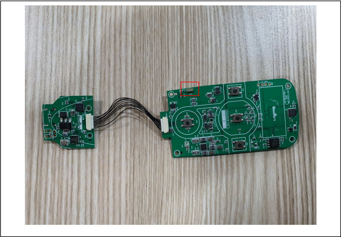
5 GHz Ant
