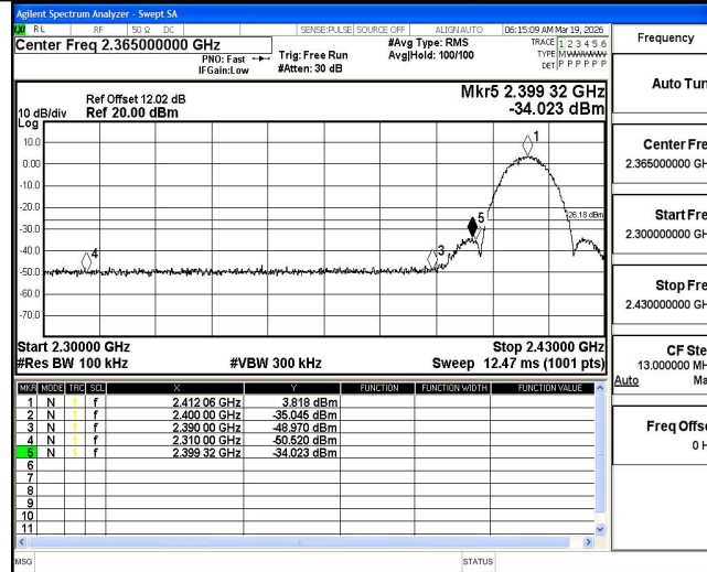
11B_Ant1_Low_2412
