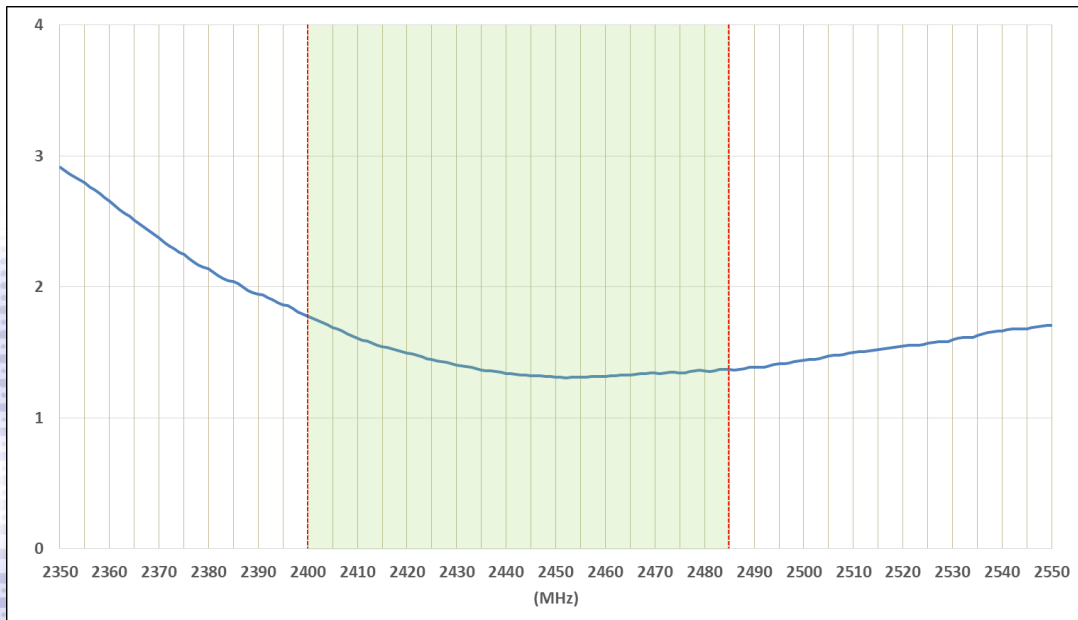
b) VSWR
