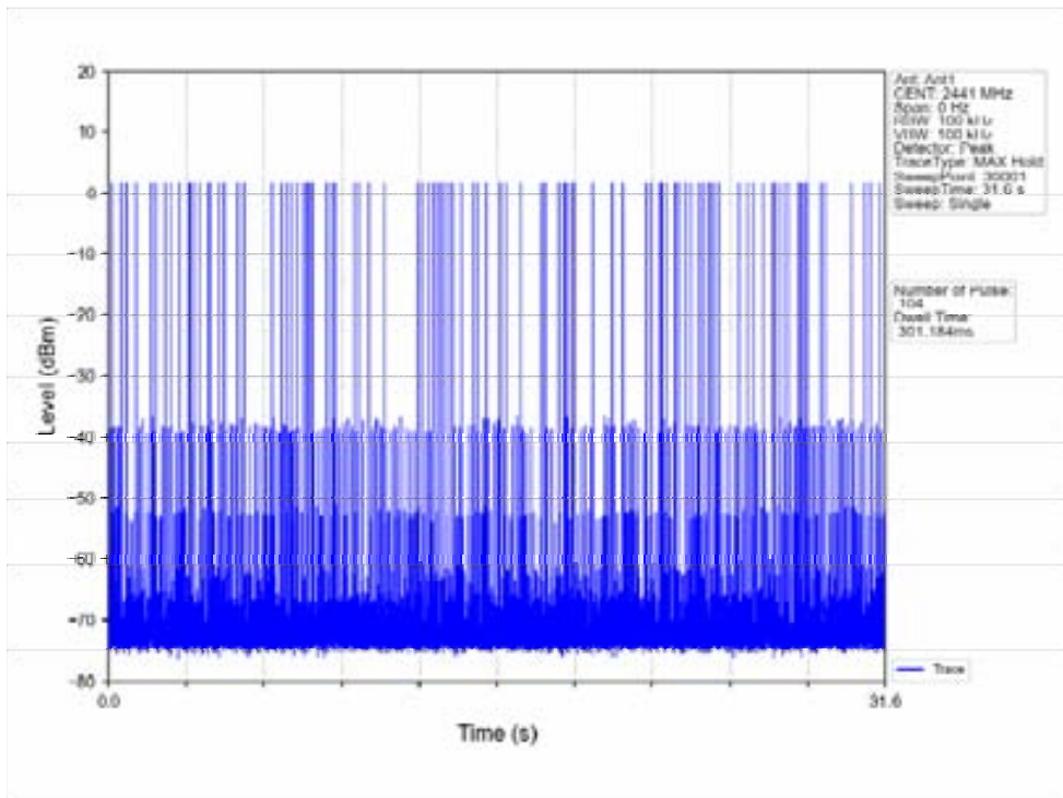
Pi/4DQPSK_2DH5_HOPP_Ant1_NTNV
