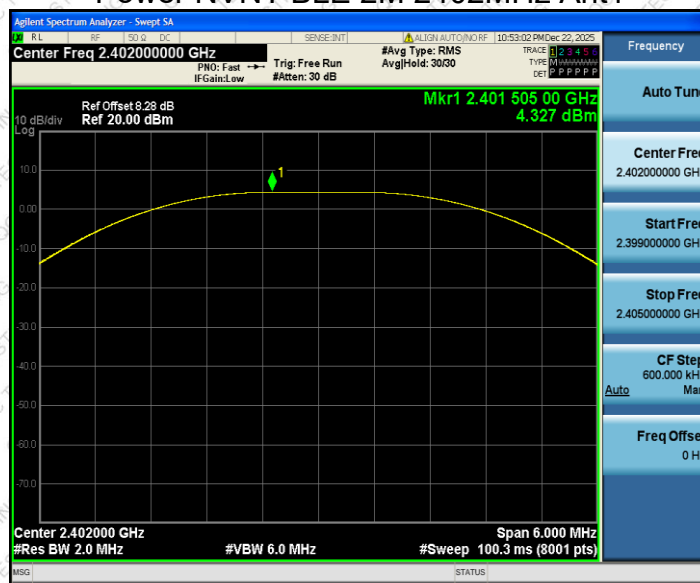
Power NVNT BLE 2M 2402MHz Ant1
