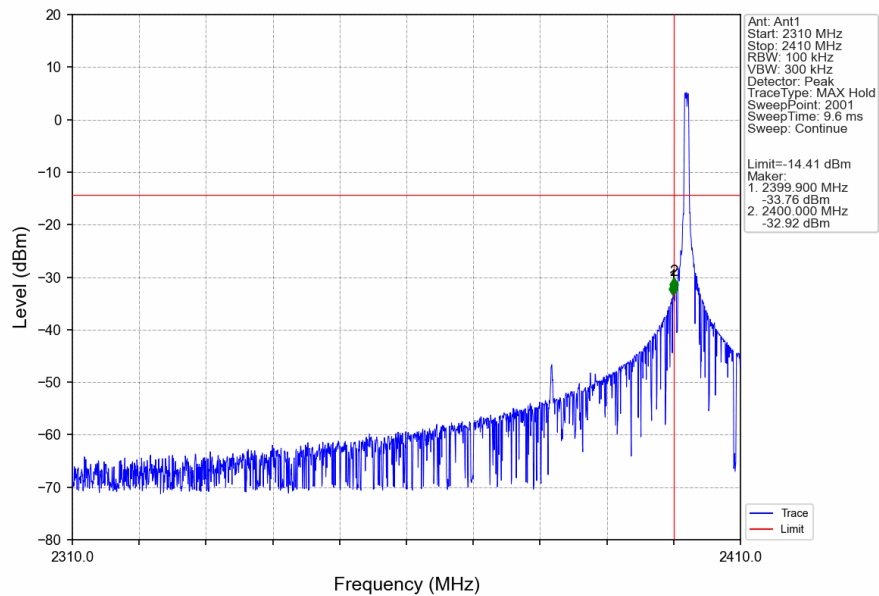
GFSK LCH 2402MHz Ant1 NTN
