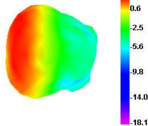
2450.000MHz
