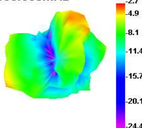
5350.000MHz
