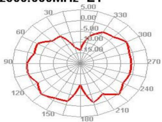
2500.000MHz E1
