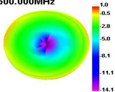
2500.000MHz
