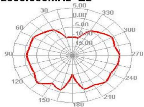
2500.000MHz E2
