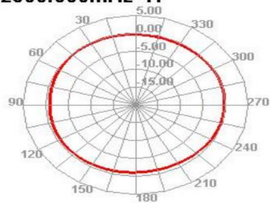
2500.000MHz H
