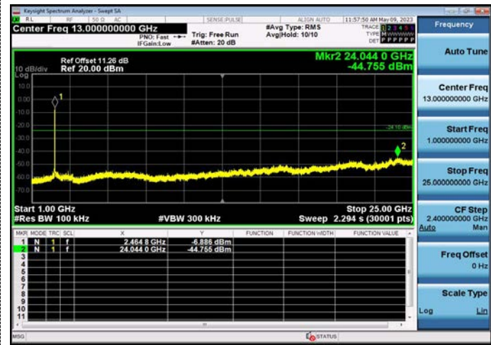
1GHz -25GHz
