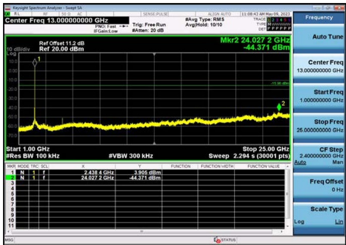
1GHz -25GHz
