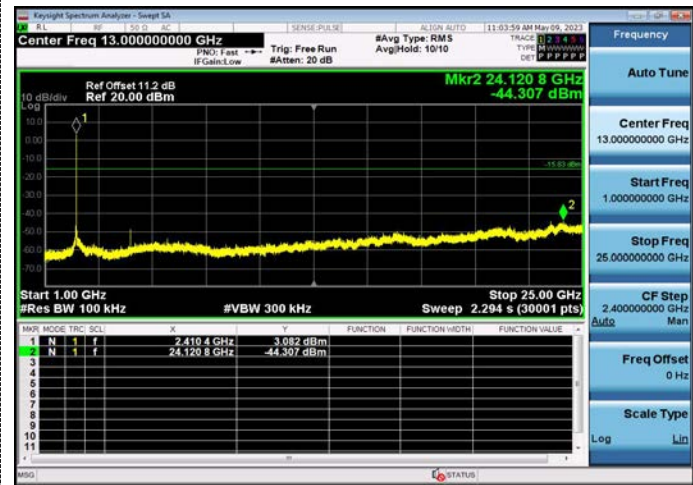
1GHz -25GHz
