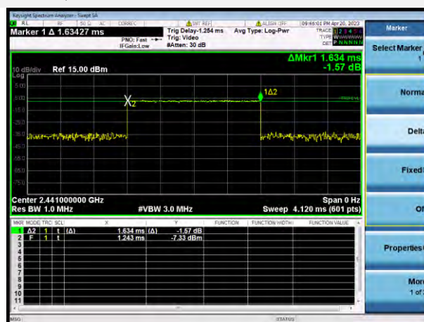
\pi/4 -DQPSK DH3
